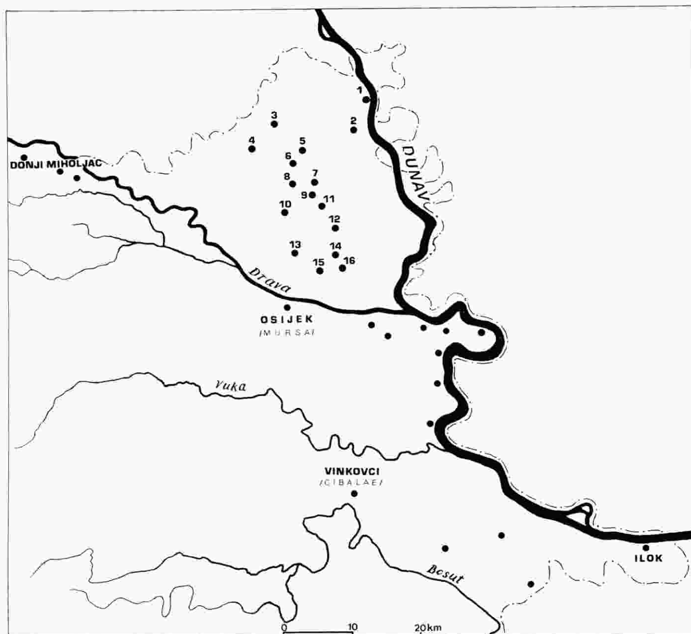
Sl. 2. Pregledna karta Limesa u Baranji. Mjerilo: 1:300.000. Crtelj: M. GREGL.
