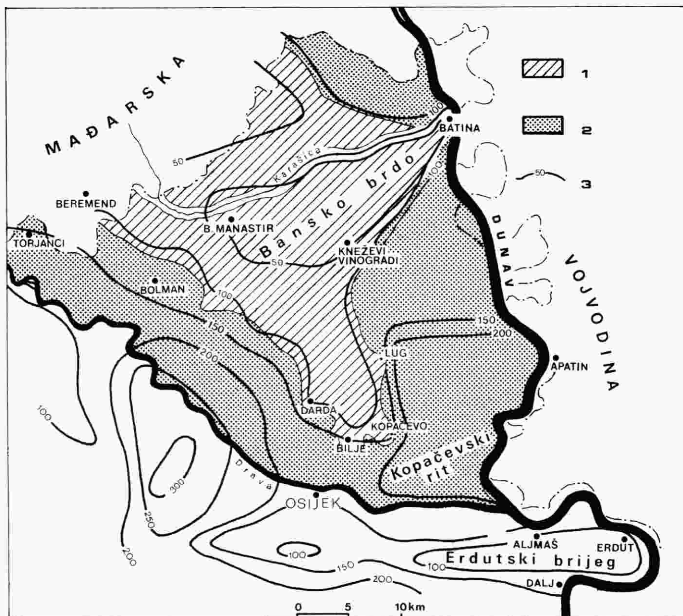
Sl. 1. Debljina kvartarnih naslaga u Baranji: 1 – Bansko brdo, lesne zaravnj i terasna nizina, 2 – polje, 3 – izobate debljina kvartarnih naslaga. Crtež: MILJENKO GREGL.
