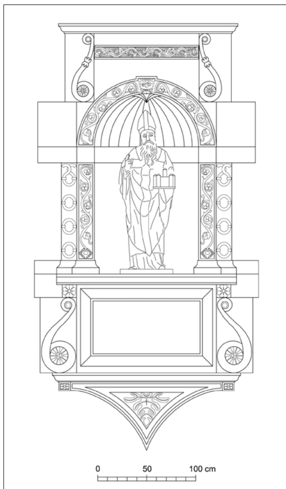
Niša na sjevernom zidu obrambenog dvorišta zapadnih vrata Dioklecijanove palače (rekonstrukcija K. Marasović)
