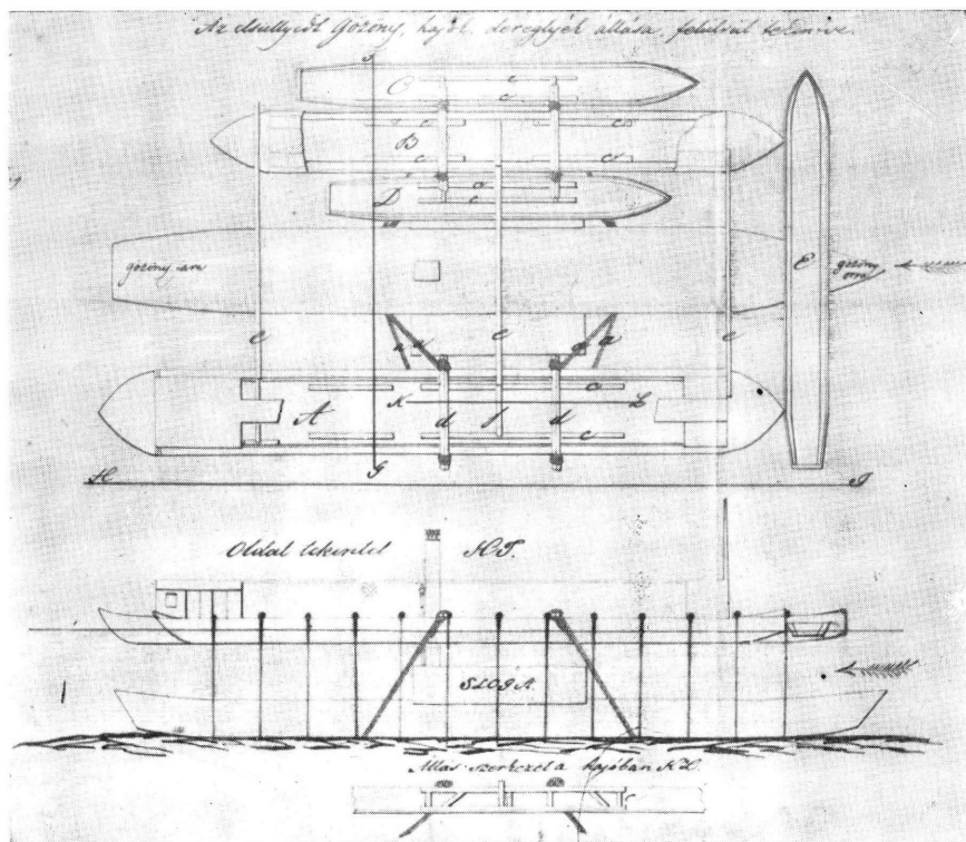
Sl. 2. Nacrt o dizanju potonulog parobroda »Sloge« iz vode. V. dok. br. 28-33.
