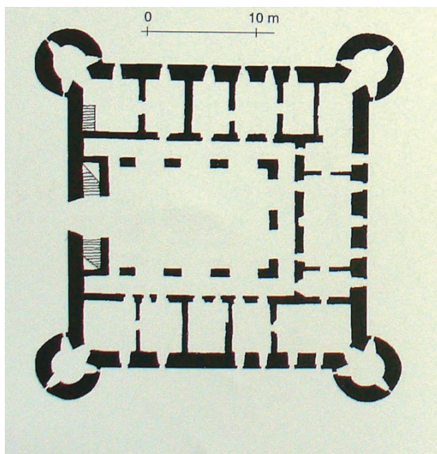
Slika 30. Cernik – tlocrt prizemlja kaštela (M. i B. Bojanić Obad Šćitaroci, Perivoji i dvorci Slavonije, Zagreb 1998)
