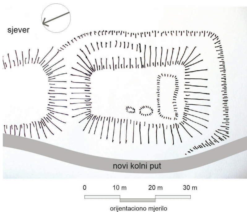
Slika 6. Tvrđić-skica tlocrta (N. Miličić, K. Regan, 2013)
