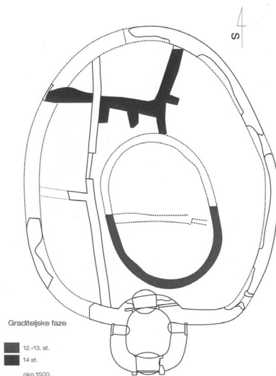
Slika 2 Gračanica-tlocrt (R. Ivanušec, Z. Horvat, M. Mihaljević, Utvrda Gračanica 2011)
