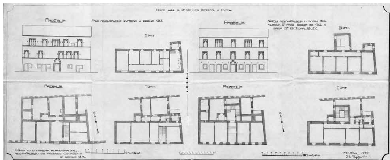
Muzej hvarske baštine, precrtani izvorni projekt rekonstrukcije donje palače Paladinić iz 1870. godine, Mostar, 1925. godine (autor: J. S. Ugojkov) / Hvar Heritage Museum, copy of the original project of reconstruction of the lower Paladinić palace 1870, Mostar 1925 (author: J. S. Ugojkov)
