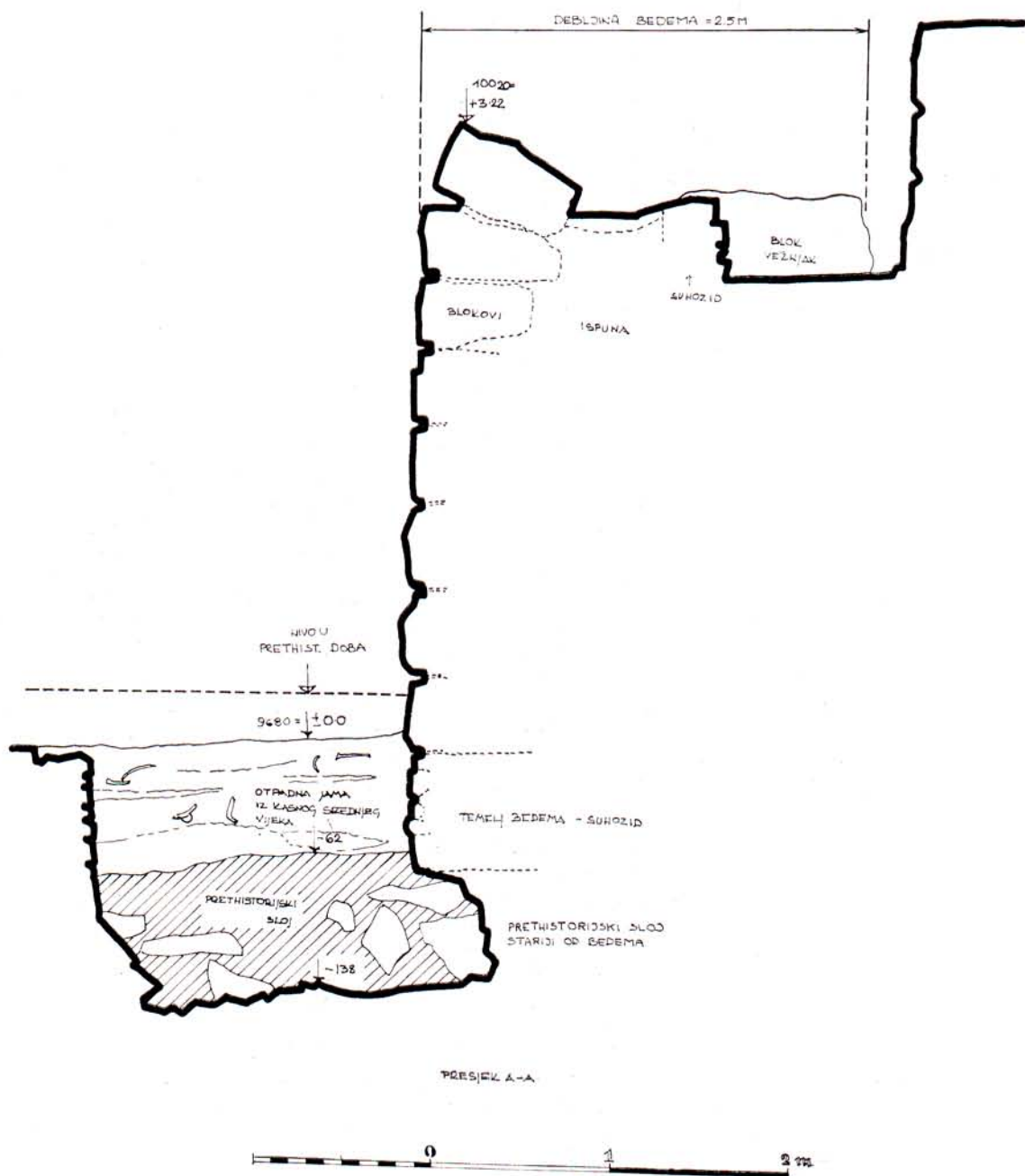
6 Presjek kroz protohistorijski bedem u zapadnoj dionici (A. F.) Section through the western Iron Age wall.
