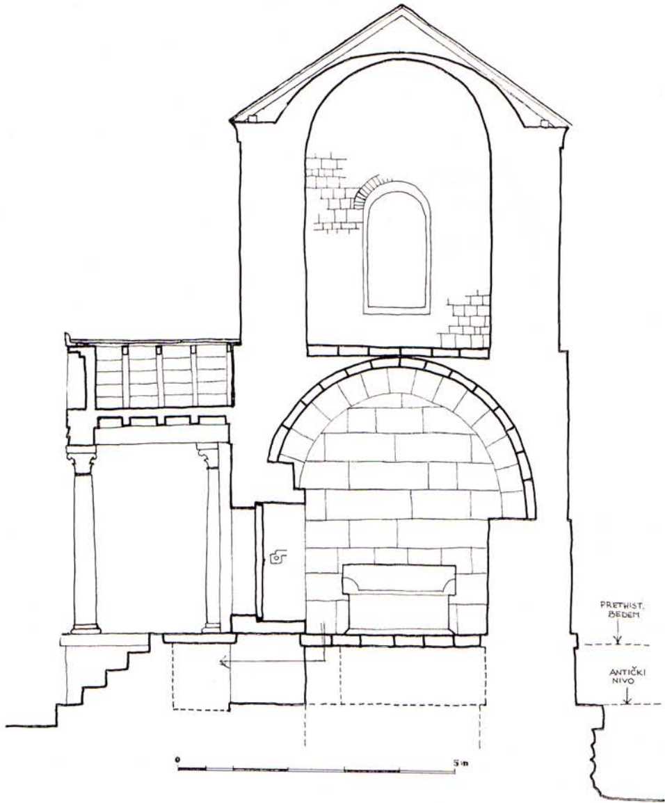
14 Presjek rekonstrukcije mauzoleja (A. Faber — Đ. Brajuka) Section of the mausoleum, reconstructed.
