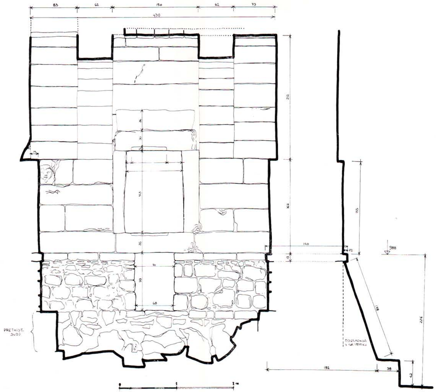
10 Presjek S—J mauzolej s pogledom na vrata cele i na pomoćni izlaz. U lijevom uglu mali reljef. (A. Faber — S. Machiedo)
