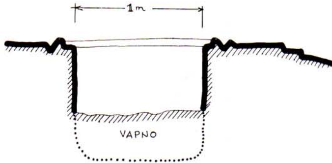
PRESJEK GROBA ③ Mj 1: 20
