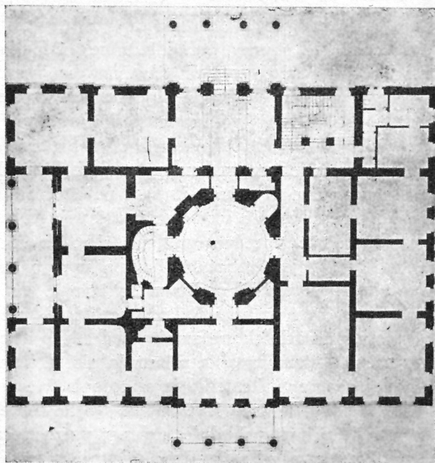
Sl. 2 — Tlocrt
