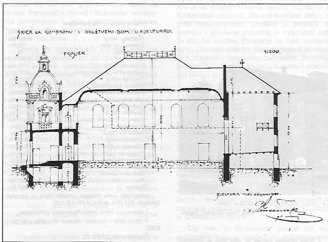
Sl. 2 - Inž. Srećko Smočinski: Presjek zgrade Sokolskog doma, skica iz 1910. godine
