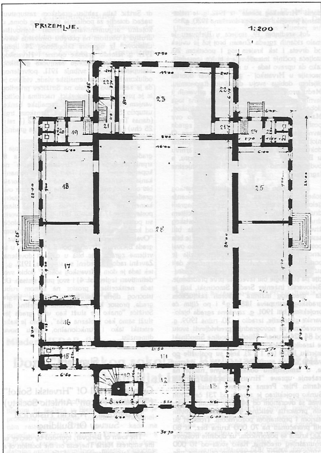
Sl. 1. - Inž. Srećko Smočinski: Tlocrt prizemlja Sokolskog doma, skica iz 1910. godine
