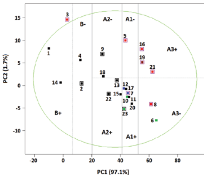
Slika 8. PCA grafikon za područja jedinica lokalne samouprave Bjelovarsko-bilogorske županije (brojevi u zagradama označuju jedinice lokalne samouprave u tablici 1)
