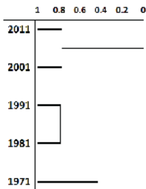
Slika 5. HCA dendrogram za varijable, tj. godine popisa stanovništva
