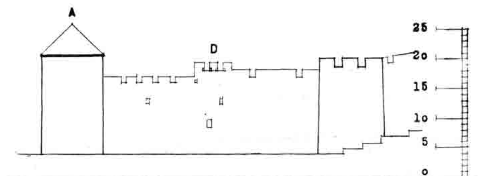
Sl. 60 — Nacrt 7a — Kaštel — XVII st. Rekonstrukcija pročelja »A«.
