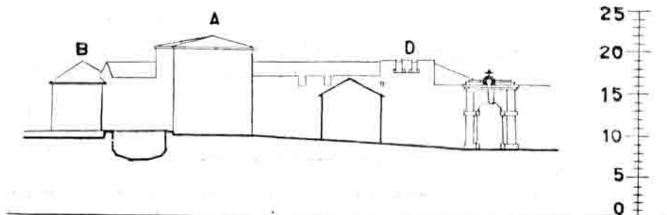
Sl. 57 — Nacrt 2a — Kaštel — prije 1896. Rekonstrukcija pročelja »A«.
