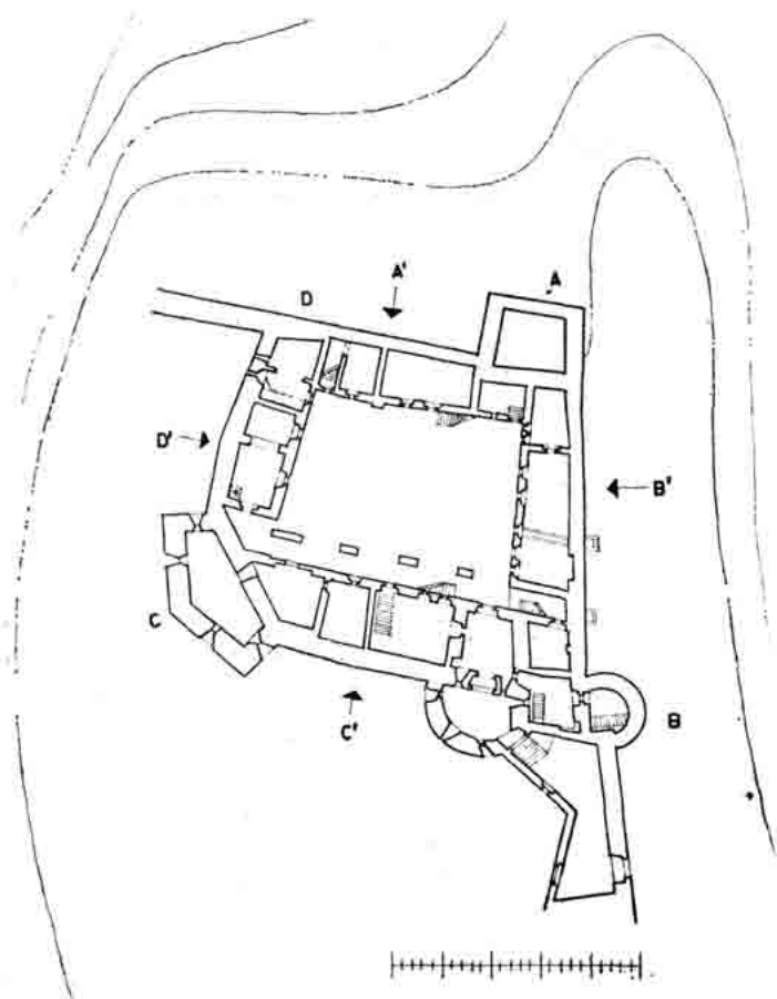
Sl. 76 — Nacrt 4e — Kaštel — prije 1763. Tlocrt prizemlja.
