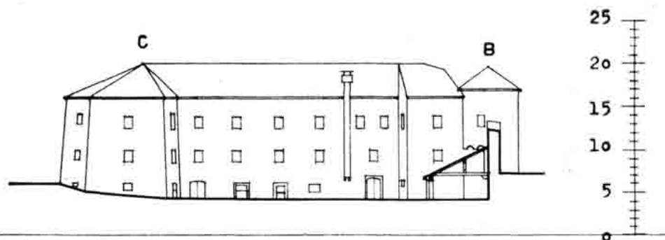
Sl. 67 — Nacrt 2c — Kaštel — prije 1896. Rekonstrukcija pročelja »C«.
