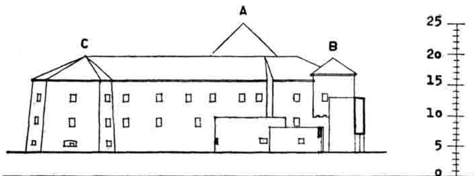
Sl. 69 — Nacrt 4c — Kaštel — prije 1763. Rekonstrukcija pročelja »C«.
