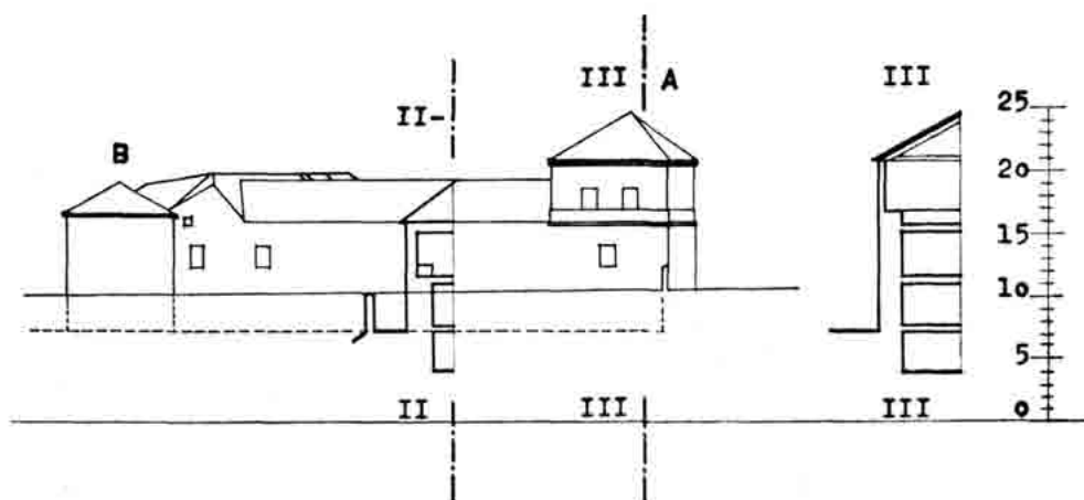
Sl. 61 — Nacrt 1b — Kaštel — današnje stanje. Pročelje »B«.
