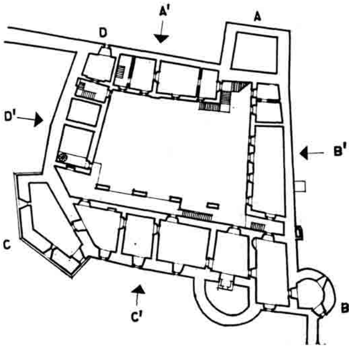
Sl. 79 — Nacrt 4f — — Kaštel — prije 1763. Tlocrt I kata.
