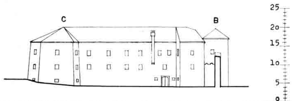
Sl. 68 — Nacrt 3c — Kaštel — iza 1763. Rekonstrukcija pročelja »C«.
