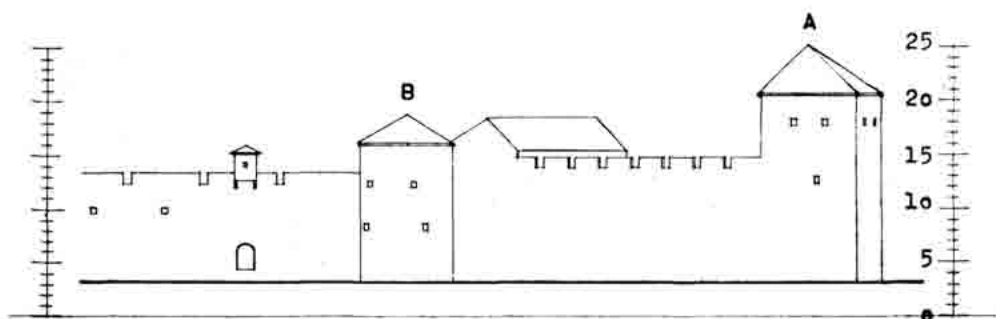
Sl. 65 — Nacrt 7b — Kaštel — XVII st. Rekonstrukcija pročelja »B«.
