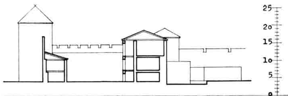
Sl. 86 — Nacrt 7e — Kaštel — XVII st. Rekonstrukcija presjeka I — I.
