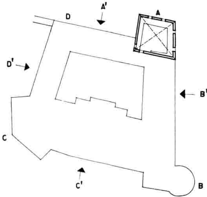
Sl. 85 — Nacrt 1h — Kaštel — današnje stanje. Tlocrt III kata.
