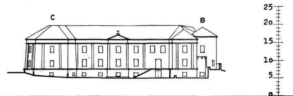
Sl. 66 — Nacrt 1c — Kaštel — današnje stanje. Pročelje »C«.
