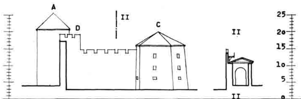
Sl. 75 — Nacrt 7d — Kaštel — XVII st. Rekonstrukcija pročelja »D«.
