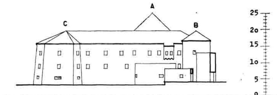
Sl. 70 — Nacrt 7c — Kaštel — XVII st. Rekonstrukcija pročelja »C«.
