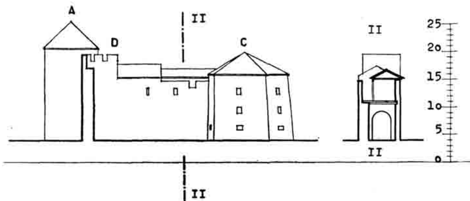
Sl. 74 — Nacrt 4d — Kaštel — prije 1763. Rekonstrukcija pročelja »D«.
