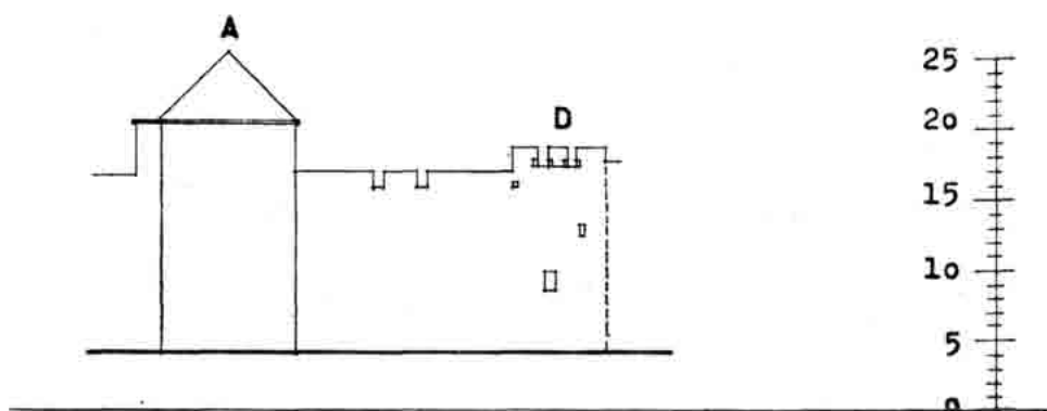
Sl. 59 — Nacrt 4a — Kaštel — prije 1763. Rekonstrukcija pročelja »A«.
