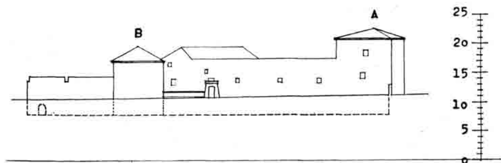
Sl. 62 — Nacrt 2b — Kaštel — prije 1896. Rekonstrukcija pročelja »B«.
