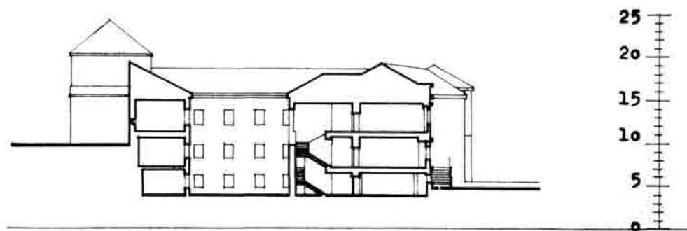
Sl. 88 — Nacrt 1f — Kaštel — današnje stanje, presjek I—I.
