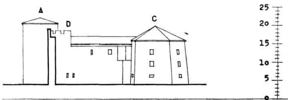
Sl. 73 — Nacrt 3d — Kaštel — iza 1763. Rekonstrukcija pročelja »D«.
