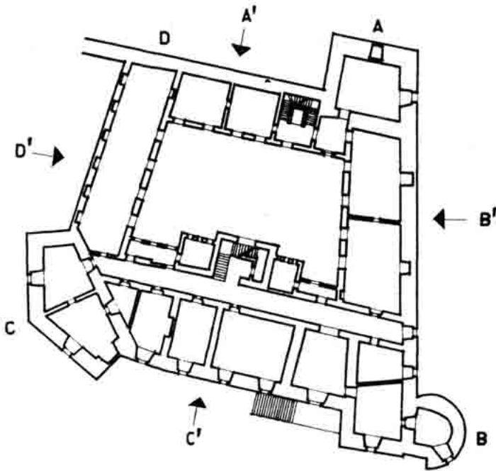
Sl. 81 — Nacrt 1f — Kaštel — današnje stanje. Tlocrt I kata.
