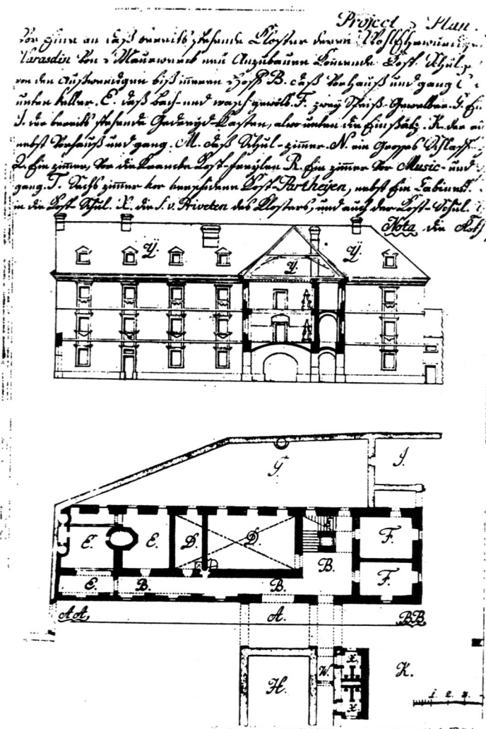
Dio plana za novogradnju uršulinskog konvikta u Varaždinu iz 1772. godine (Foto: Ivan Pančoka)
