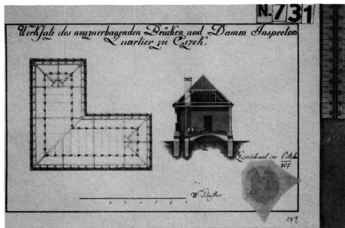
153. Plan stana inspektora mosta i nasipa na Dravi kod Osijeka, 1807. g.
