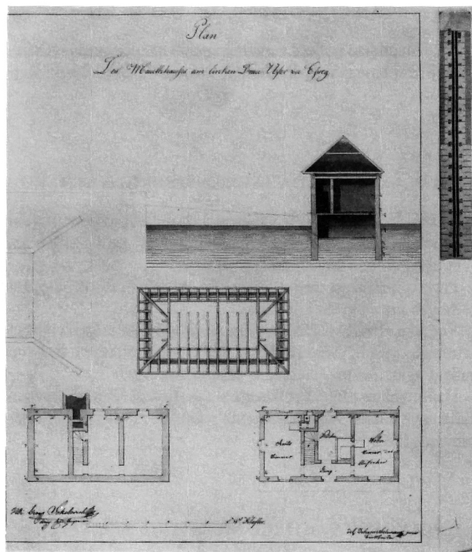
158. Plan zgrade mitnice na lijevoj obali Drave kod Osijeka, zidarski majstor Johannes Schmauss Junior, 1826. g.
