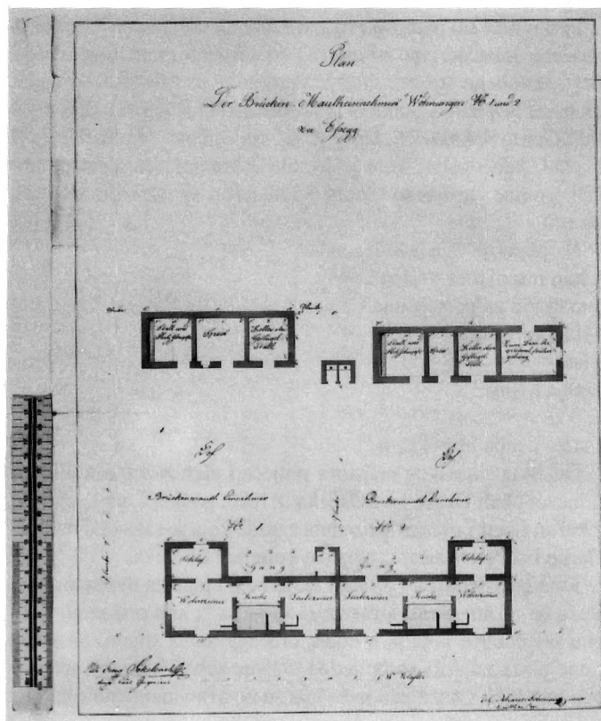
159. Plan zgrade za stanove mitničara u Osijeku, zidarski majstor Johannes Schmauss Junior, 1826. g.
