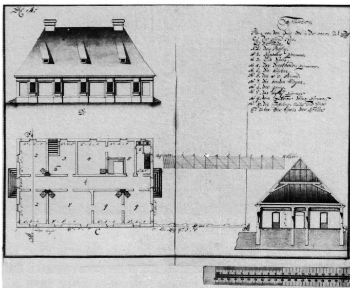
152. Plan za župni dvor u Gornjem gradu u Osijeku, zidarski majstor Anton Hautmann, 1792. g.
