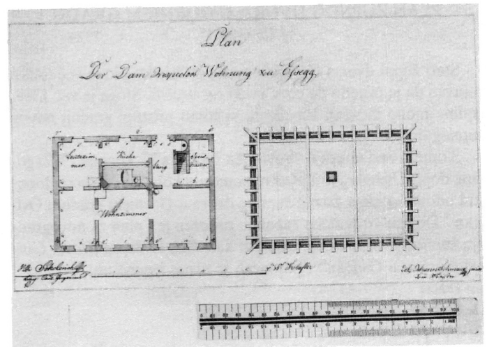
160. Plan stambene kuće za inspektora nasipa u Osijeku, zidarski majstor Johannes Schmauss Junior, 1826. g.
