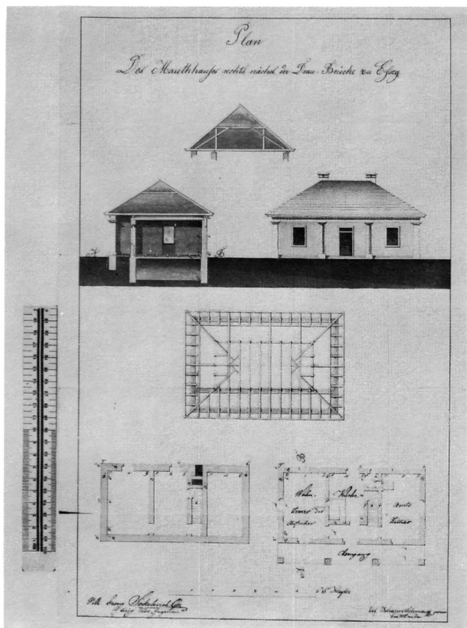
161. Plan stambene zgrade mitnice na desnoj obali Dravskoga mosta kod Osijeka, zidarski majstor Johannes Schmauss Junior, 1826. g.
