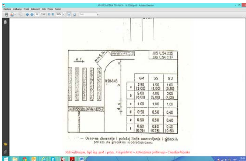
Slika 4. Osnovne dimenzije i položaj pješačkih prijelaza na gradskim prometnicama
