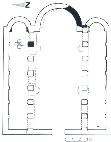
Rekonstrukcija tlocrta ranohrišćanske bazilike sv. Marije sa krstionicom u sjevernom brodu (isprekidanom linijom označen gabarit romaničke crkve sv. Marije iz 1221. godine).
