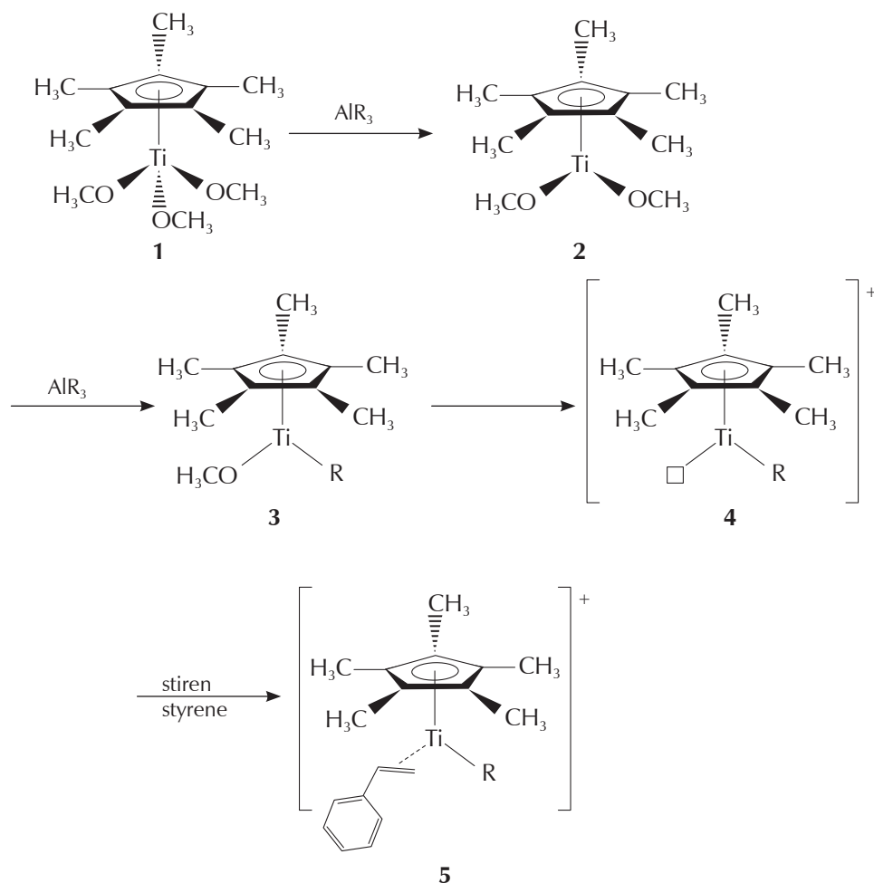
Slika 14 – Mehanizam nastajanja sindiotaktnog polistirena polimerizacijom stirena uz metalocenski katalizator, pentametilciklopentadieniltitanijev trimetoksid 70
