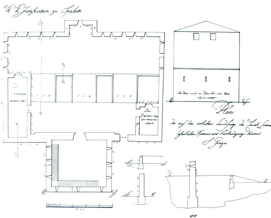
Nacrti utvrde u Sućurju iz 1822. godine (Ratni arhiv, Beč)
