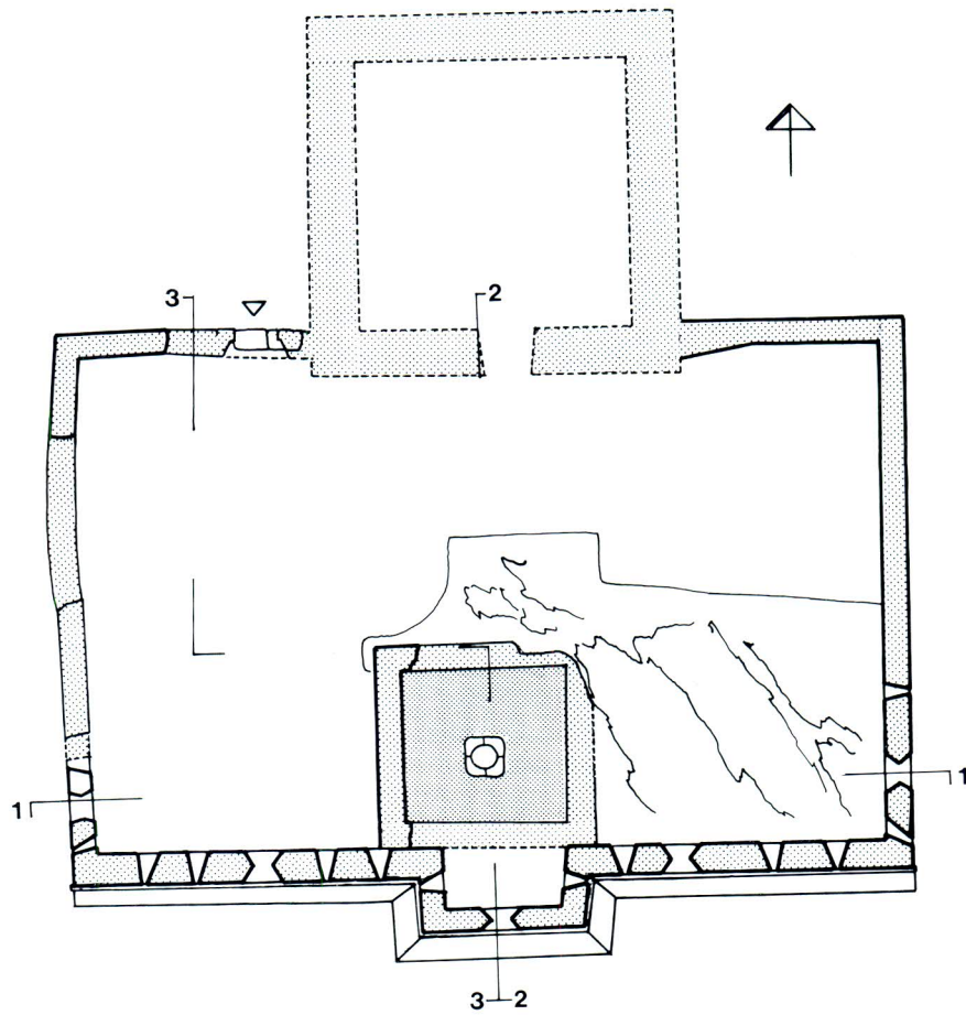
Tlocrt utvrde u Sućurju
