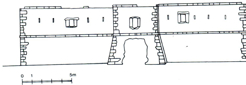
Južno pročelje
