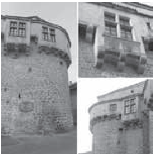
Kaštel, detalji – konzole ophodnog puta polukružne kule
