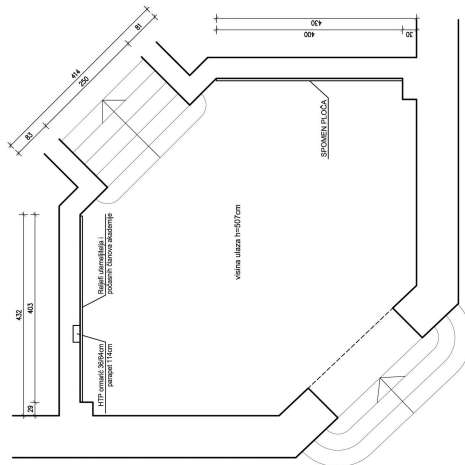
TLOCRT
