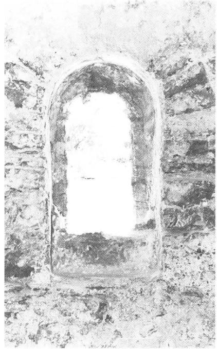
Vanjština i unutrašnjost prozora apside s ugrađenom tranzenom
