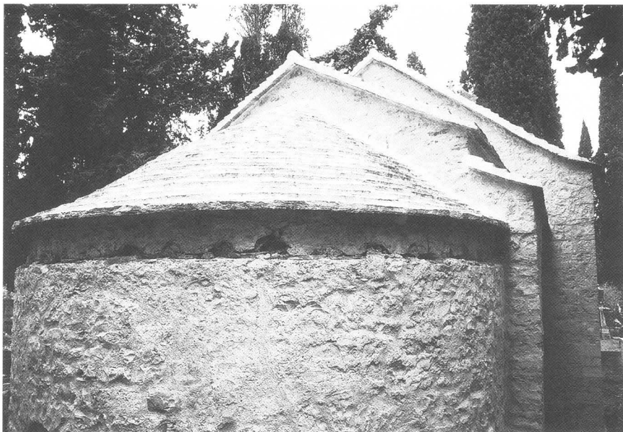
Apsida ranokršćanske crkve s pokrovom od tegula i srednjovjekovnim nadozidom
