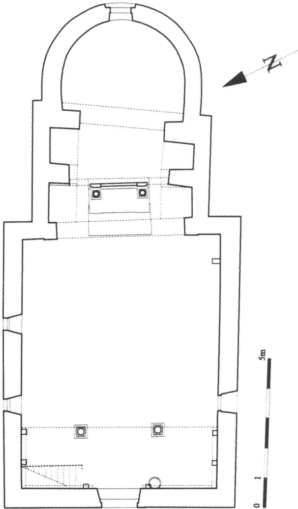
Tlocrt crkve Gospe od Utjehe (ranije Sv. Stjepan), postojeće stanje prije zaštitnih radova
