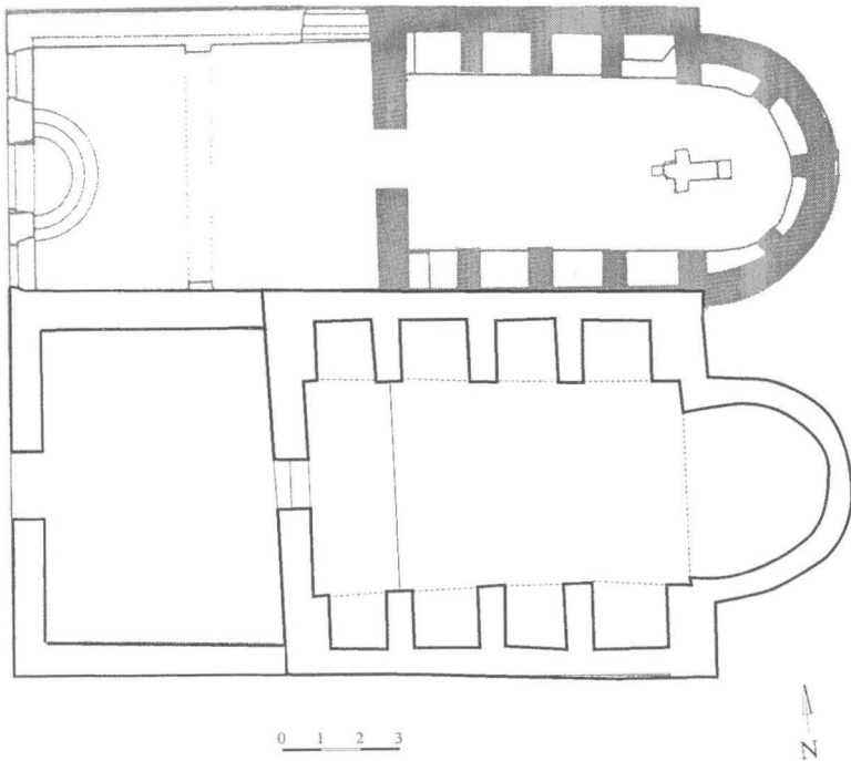
Tlocrt crkava sv. Marije i sv. Ivana u Starom Gradu u 11. st.
