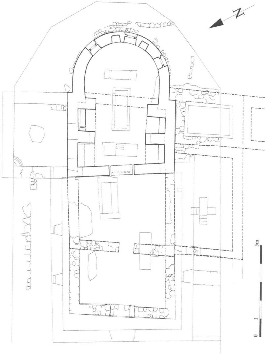
Tlocrt ranosrednjovekovne crkve sv. Stjepana u Pučišćima
