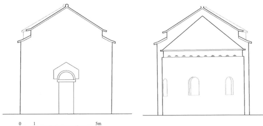
Rekonstrukcija zapadnog i istočnog pročelja crkve sv. Stjepana u Pučišćima
