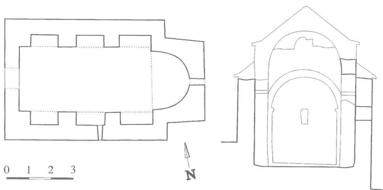
Tlocrt i presjek ruševina crkve na Sušcu (prema I. Fiskoviću)
