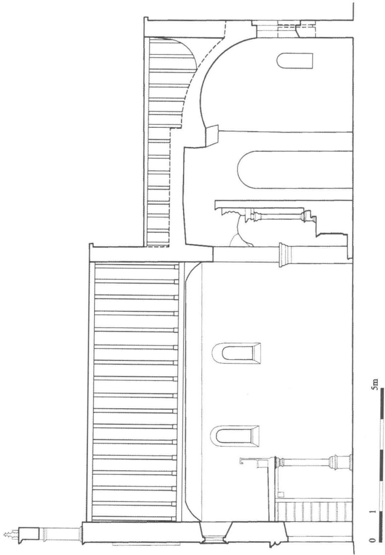
Uzdužni presjek crkve sv. Stjepana u Pučišćima, snimak postojećeg stanja prije istraživanja
