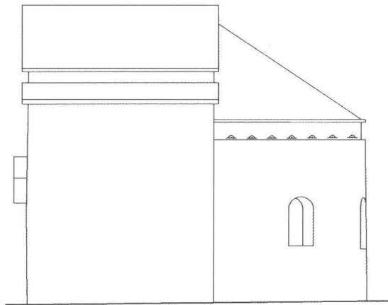
Tlocrt i pogled na južno pročelje ranosrednjovjekovne crkve sv. Stjepana u Pučišćima
