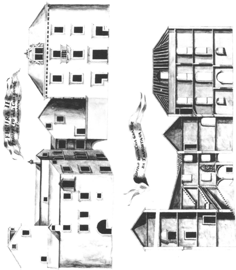
Nacrti palača Garagnin - izgled i presjeci, Muzej grada Trogira
