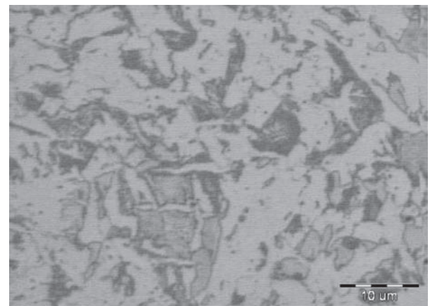
e) Microstructure
