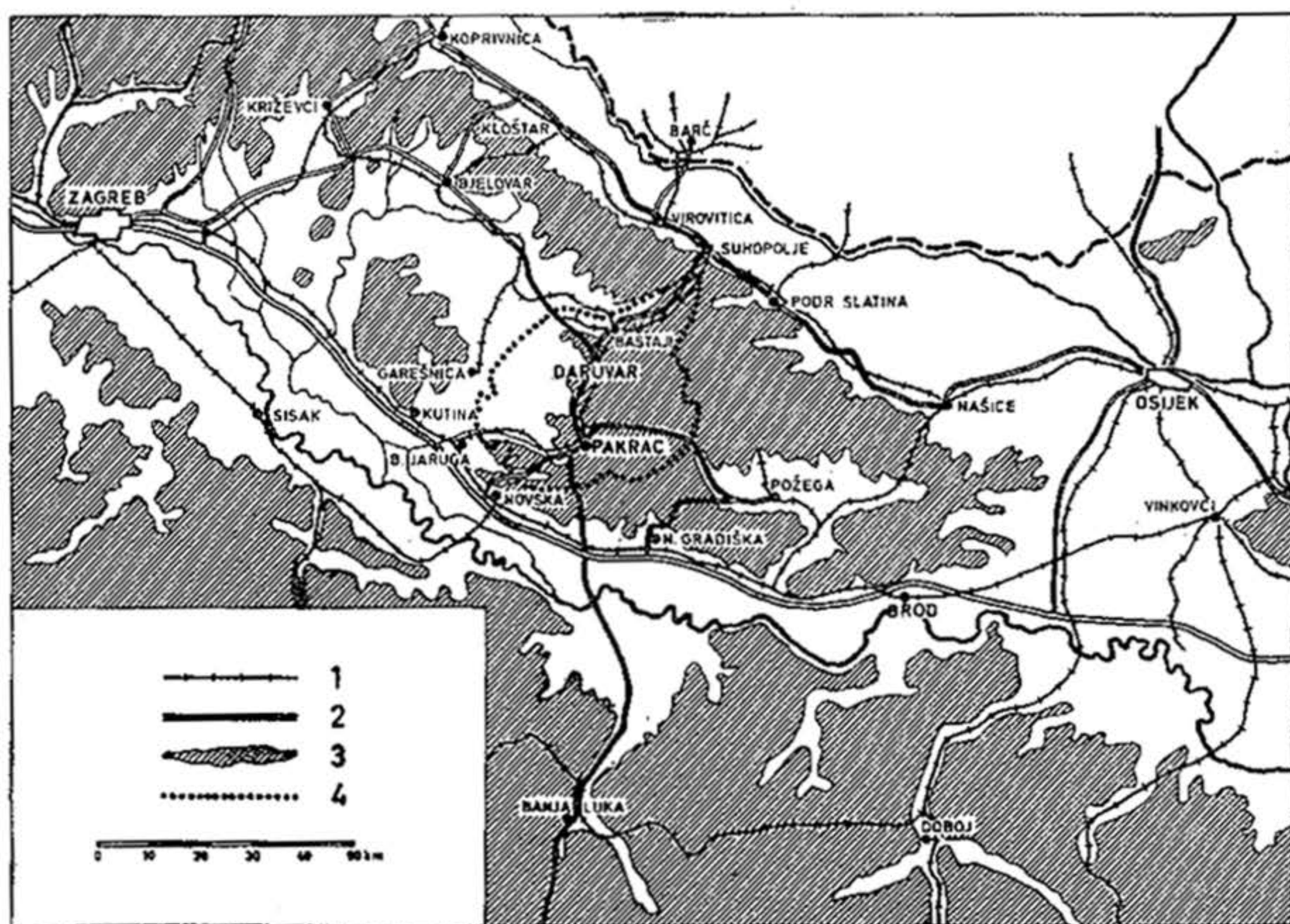
Sl. 1 Topografska karta daruvarsko-pakračkoga kraja. 1 — željezničke pruge, 2 — važnije ceste, 3 — apsolutne visine iznad 200 m, 4 — granica kraja
