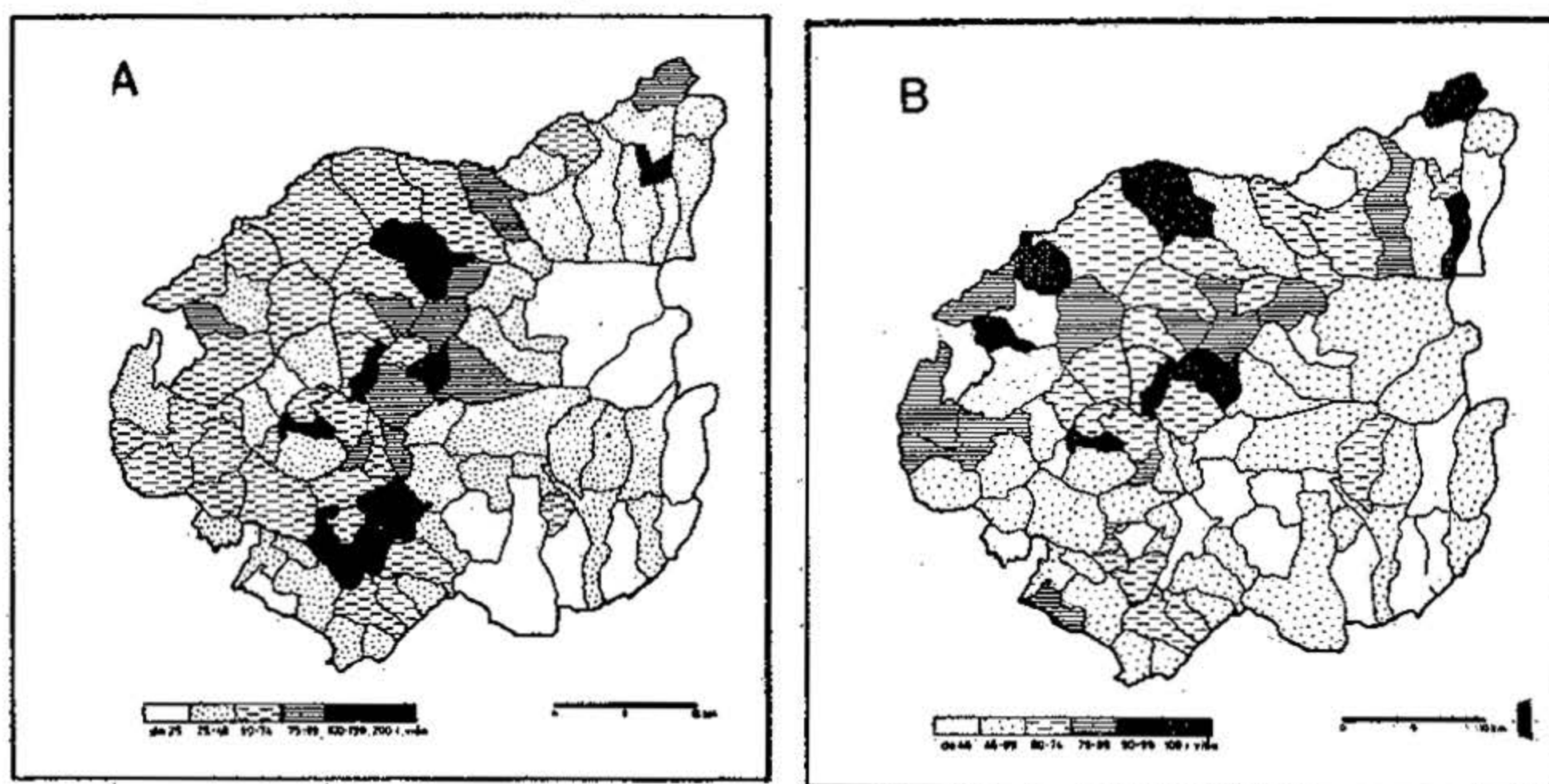
Sl. 6 A) Opća relativna gustoća u katastarskim općinama daruvarsko-pakračkoga kraja 1961. g. B) Poljoprivredna gustoća u katastarskim općinama daruvarsko-pakračkoga kraja 1961. g. C) Ratarska gustoća u katastarskim općinama daruvarsko-pakračkoga kraja 1961. g.
