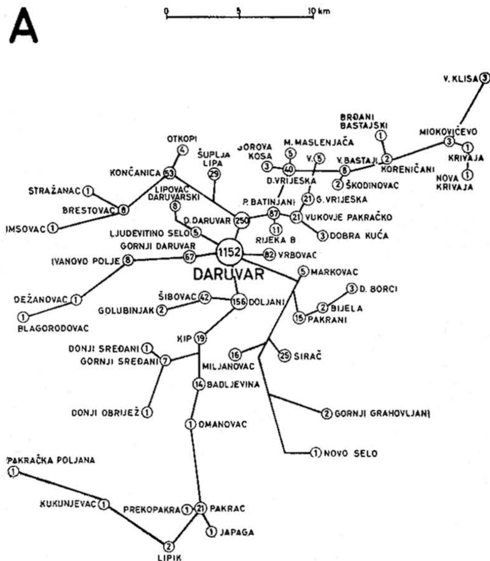
Sl. 12. A) Dnevni migranti u Daruvar iz daruvarsko-pakračkoga kraja 1961.g. Fig. 12. A) Daily commuters to Daruvar from the Daruvar-Pakrac area in 1961.
