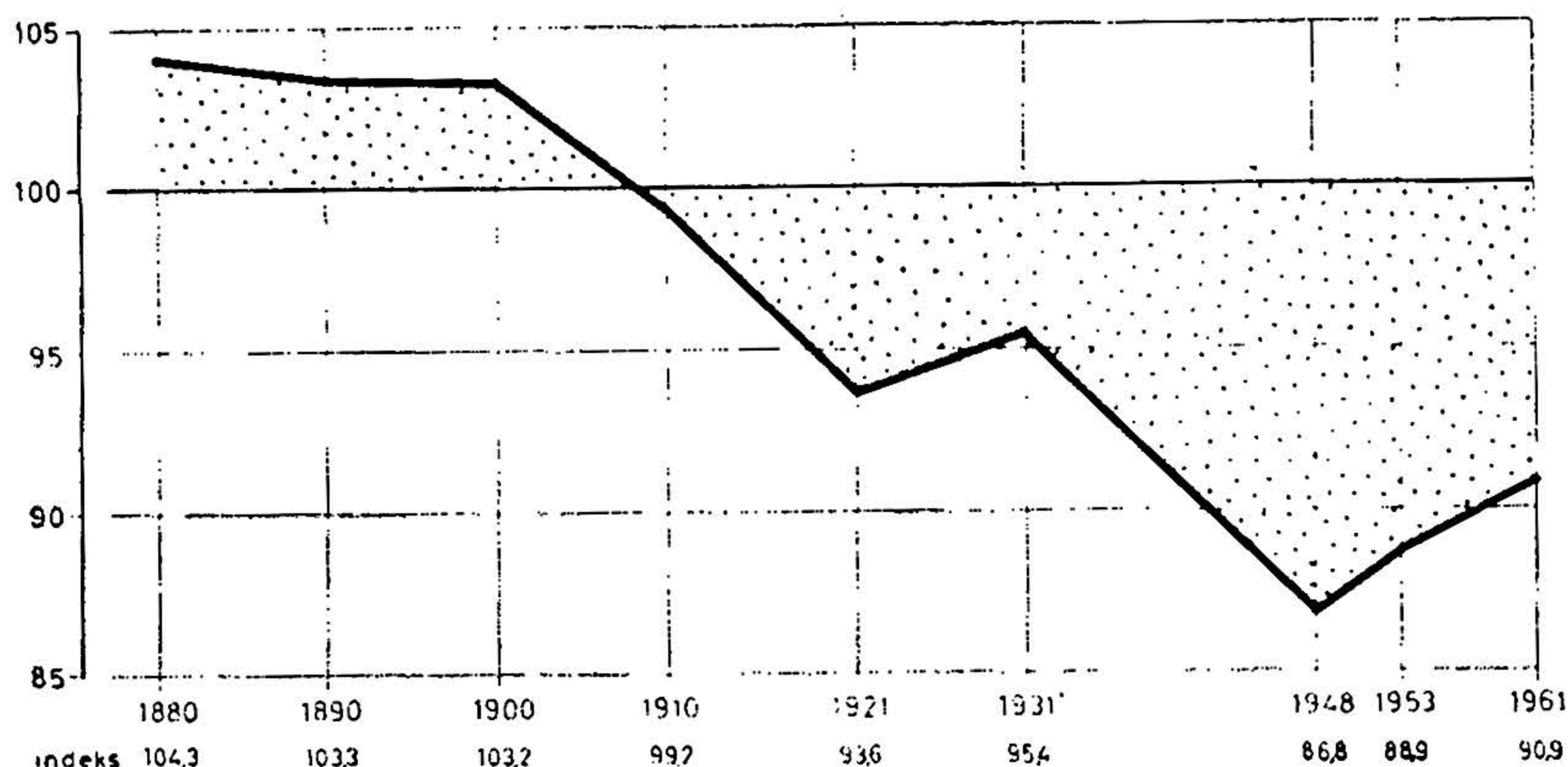
Sl. 7 Odnos broja muškaraca i žena u daruvarsko-pakračkome kraju od 1880. do 1961. g. (Broj muškaraca na 100 žena.)
