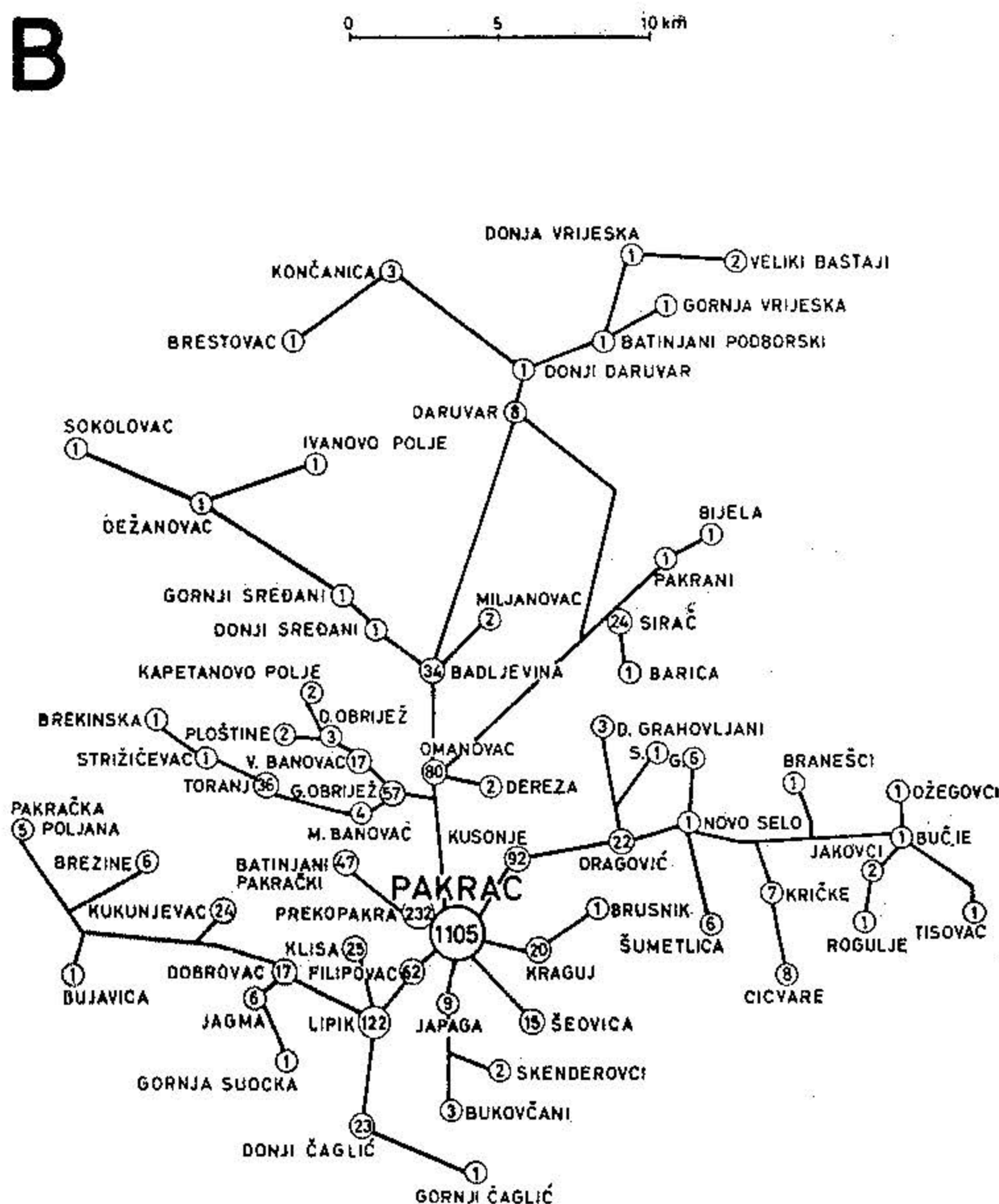
Sl. 12. B) Dnevni migranti u Pakrac iz daruvarsko-pakračkoga kraja 1961. g. Fig. 12. B) Daily commuters to Pakrac from the Daruvar-Pakrac area in 1961.
