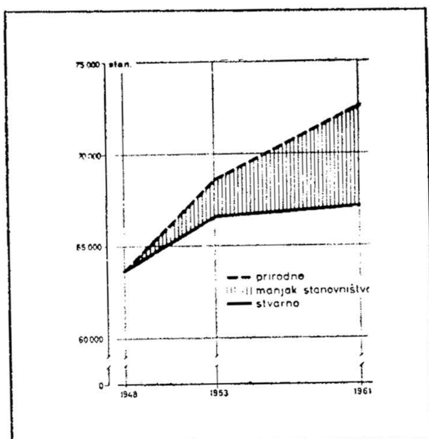
Sl. 5 Razlika između popisima utvrđenog i prirodnog kretanja broja stanovnika daruvarsko-pakračkoga kraja od 1948. do 1961. g.
