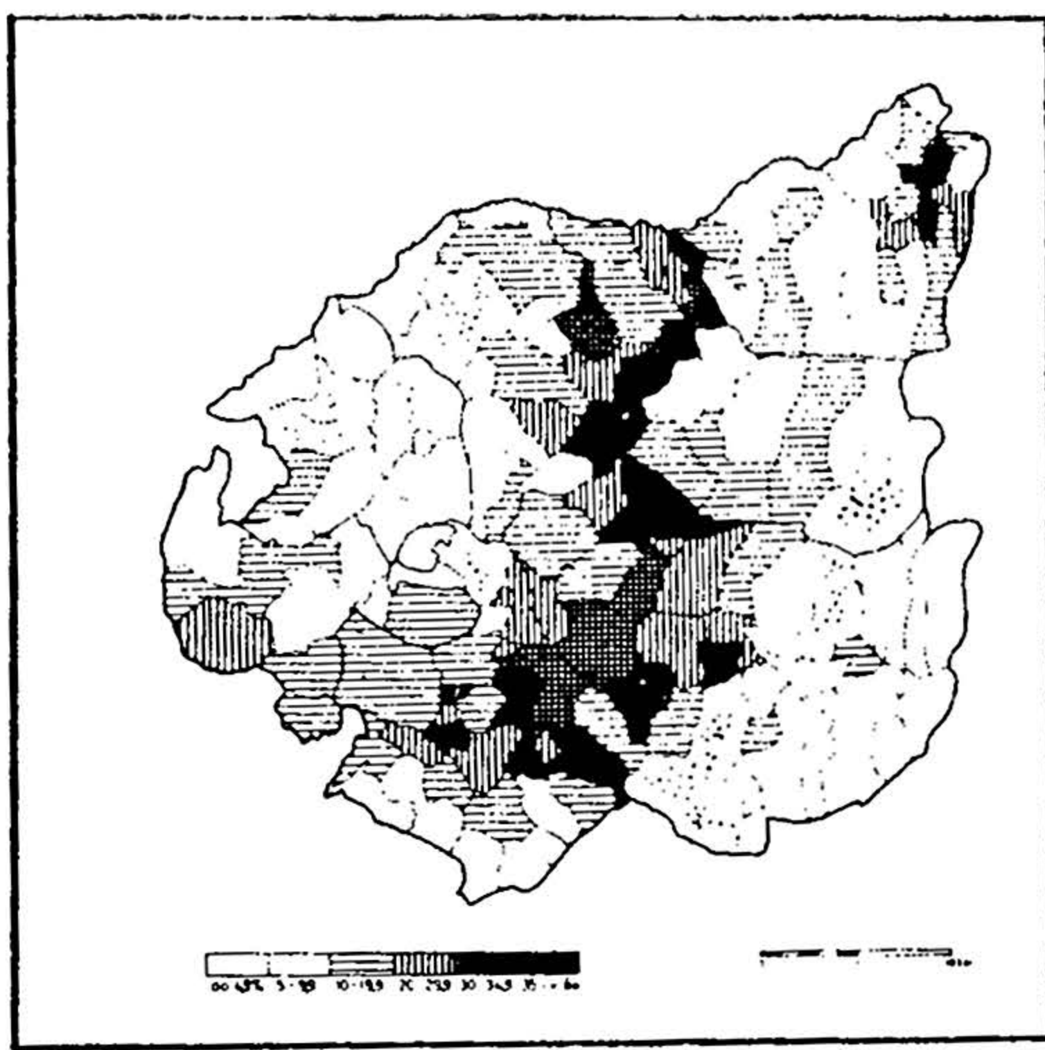
Sl. 8 Udio aktivnog stanovništva u naseljima daruvarsko-pakračkoga kraja u grupi sekundarnih gospodarskih djelatnosti 1961.g. Fig. 8. Share of gainfully employed population in places of the Daruvar-Pakrac area in the group of secondary economical activities in 1961.
