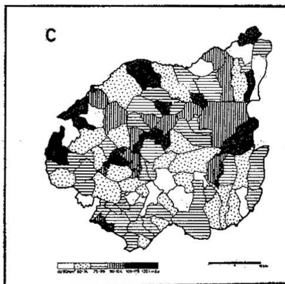
Sl. 6 A) Opća relativna gustoća u katastarskim općinama daruvarsko-pakračkoga kraja 1961. g. B) Poljoprivredna gustoća u katastarskim općinama daruvarsko-pakračkoga kraja 1961. g. C) Ratarska gustoća u katastarskim općinama daruvarsko-pakračkoga kraja 1961. g.
