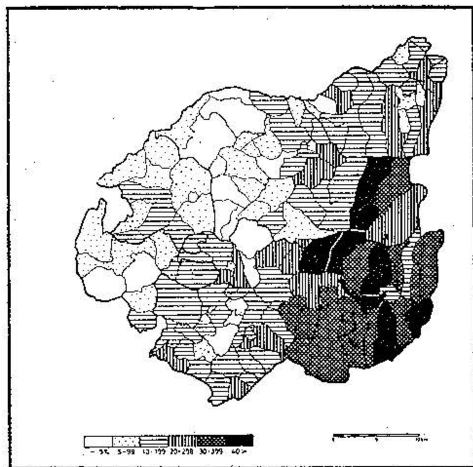
Sl. 9. Udio nepismenih među stanovništvom starijim od 10 godina u naseljima daruvarsko-pakračkoga kraja 1961. g.
