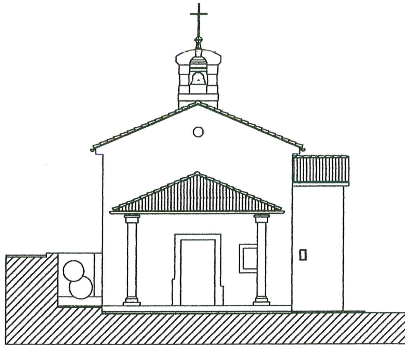
Sl. 1. Pročelje crkvice sv. Ane
