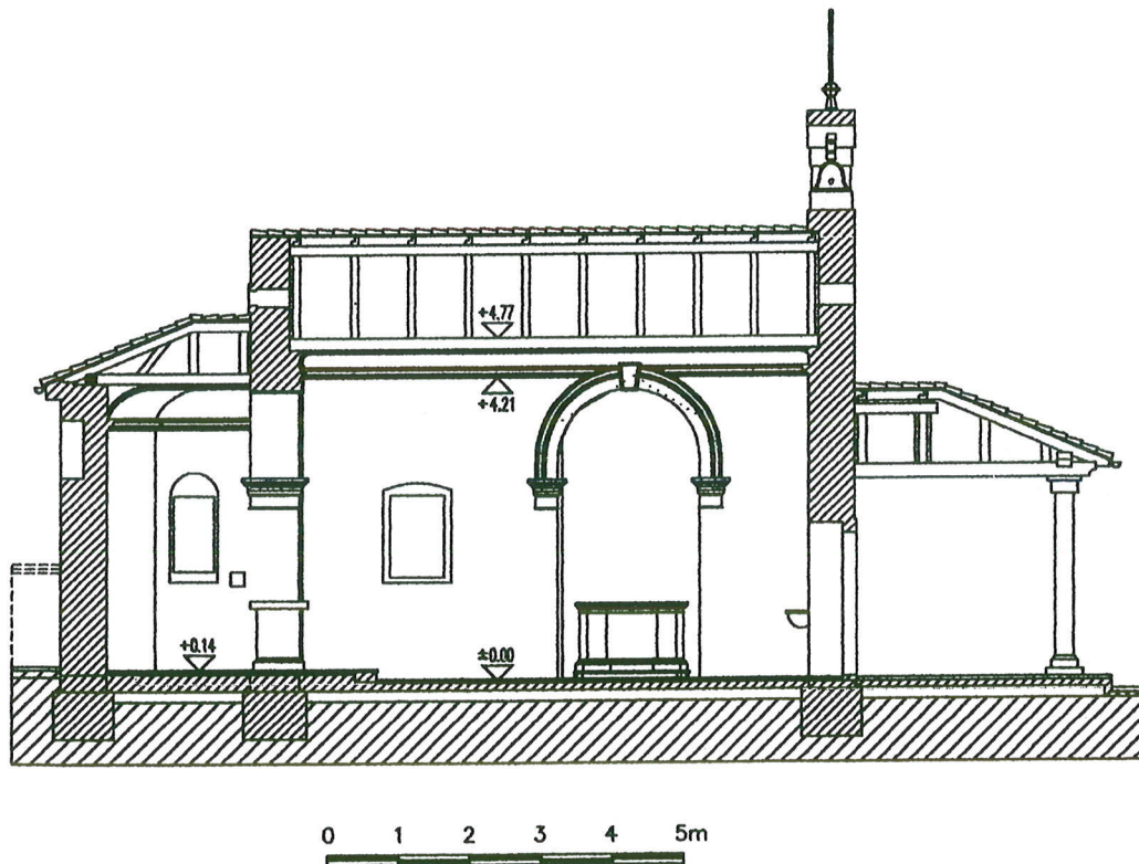
Sl. 1. Poprečni presjek apside crkvice sv. Ane
