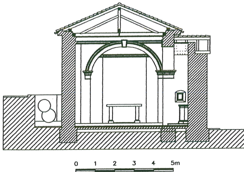
Sl. 1. Poprečni presjek apside crkvice sv. Ane
