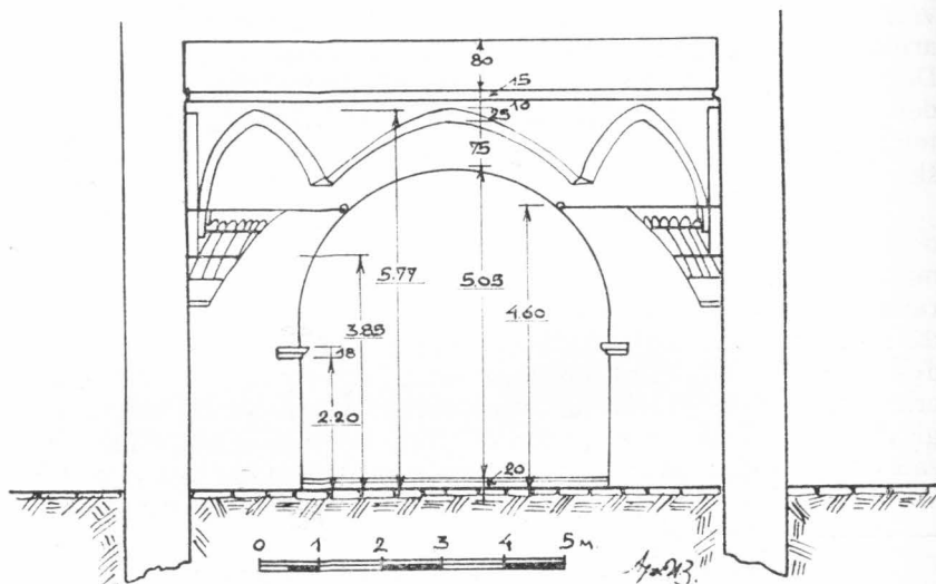
34. Presjek drniške džamije
