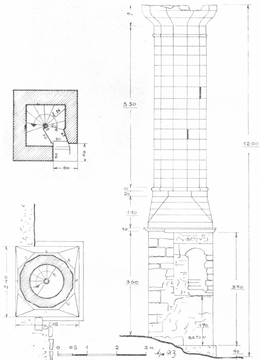
1. Nacrt minareta u Drnišu
