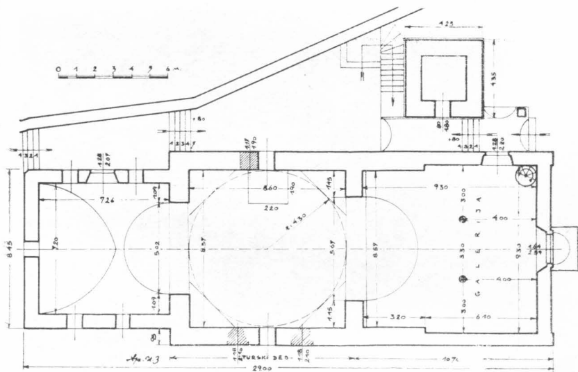
35. Tloris drniške džamije
