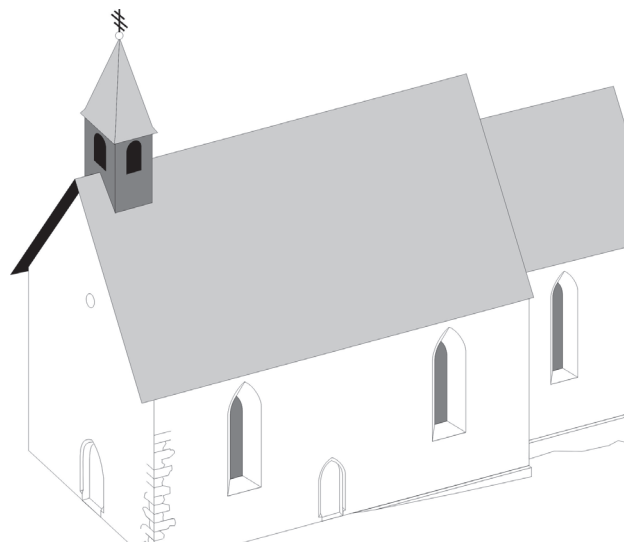
2. Prikaz izgleda kapele svetog Andrije Apostola u Kamešnici nakon izgradnje 1377., rekonstrukcija na bazi očuvanog stanja i nalaza. / Chapel of St. Andrew the Apostle in Kamešnica after 1377, reconstruction based on current state and archeological discoveries.
