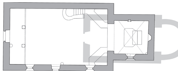
2. Prikaz izgleda kapele svetog Andrije Apostola u Kamešnici nakon izgradnje 1377., rekonstrukcija na bazi očuvanog stanja i nalaza. / Chapel of St. Andrew the Apostle in Kamešnica after 1377, reconstruction based on current state and archeological discoveries.
