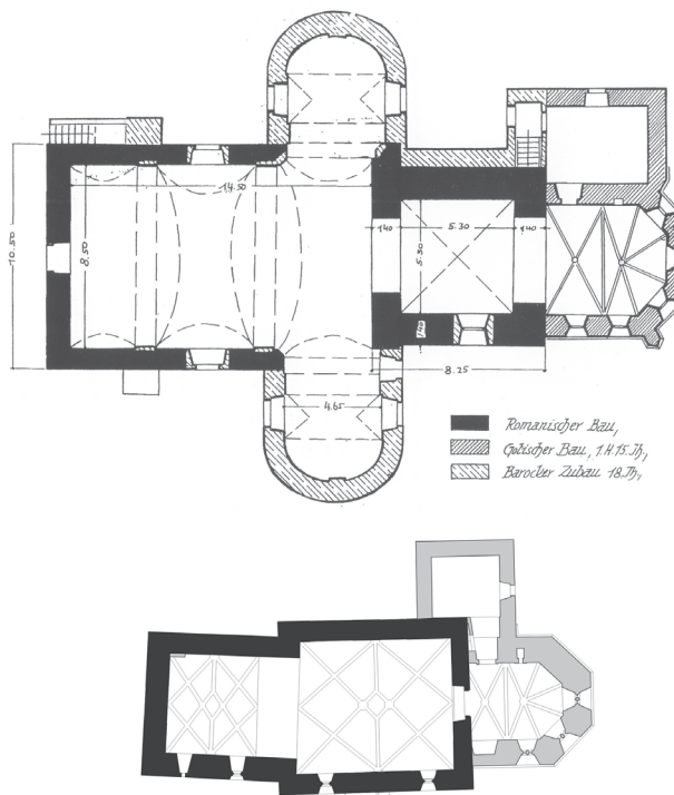
18. Usporedba prostornog razvoja župne crkve svetog Jurja u St. Georgen ob Judenburg (Prema: Pfarrkirche St. Georgen ob Judenburg , 2000., str. 9) i crkve svetog Jurja u Belec. Nacrti su u mjerilu! / Comparison of the spatial development of St. George in Belec, and of St. George in St. Georgen ob Judenburg (after: Pfarrkirche St. Georgen ob Judenburg , 2000., p. 9) (same scale).
