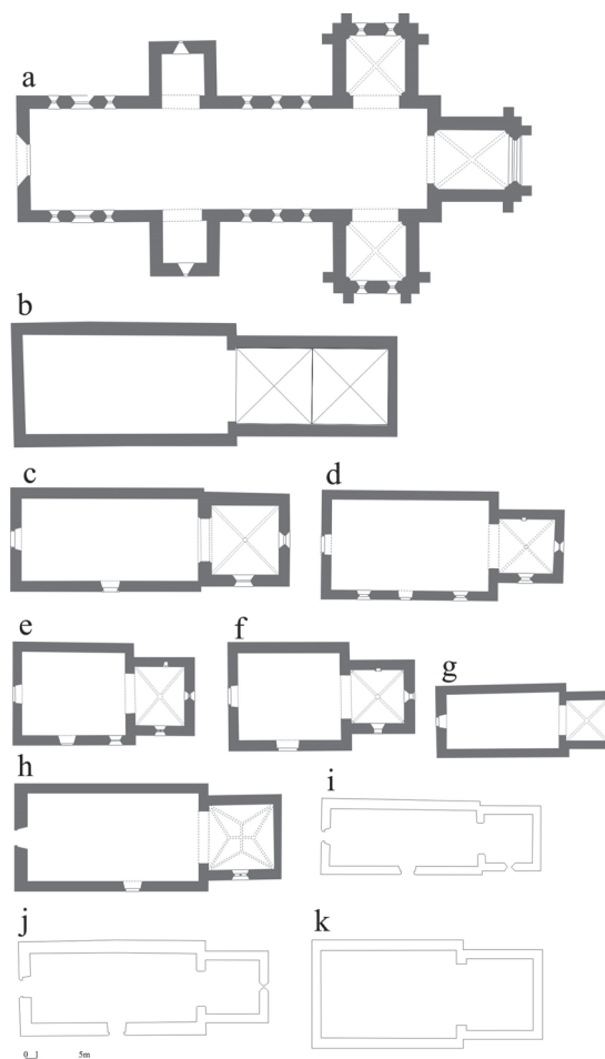
Lijevo / Left: 21. Prostorni razvoj Dominikanske crkve svete Magdalene u Čazmi kroz dvije romaničke etape. Prema: [Sveti trag – 1994.], str. 129 / Two Romanesque phases of St. Magdalene in Čazma. After: [Sveti trag – 1994.], p. 129
