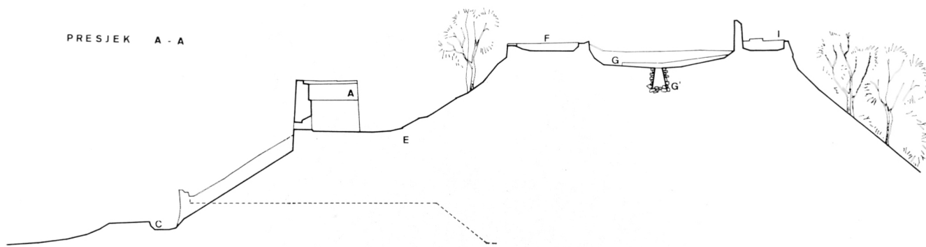
2 Presjek A—A starog grada Vitunja (arh. snimak Gvozdanović S.)
