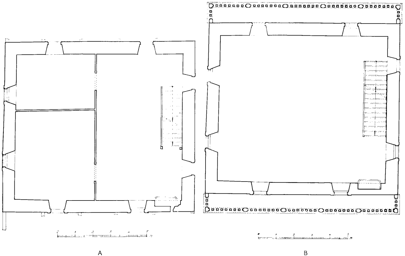
KAŠTEL CIPICO U KAŠTEL NOVOM, TLOCRT II. KATA: A — Postojeće stanje, B — Projekt.
