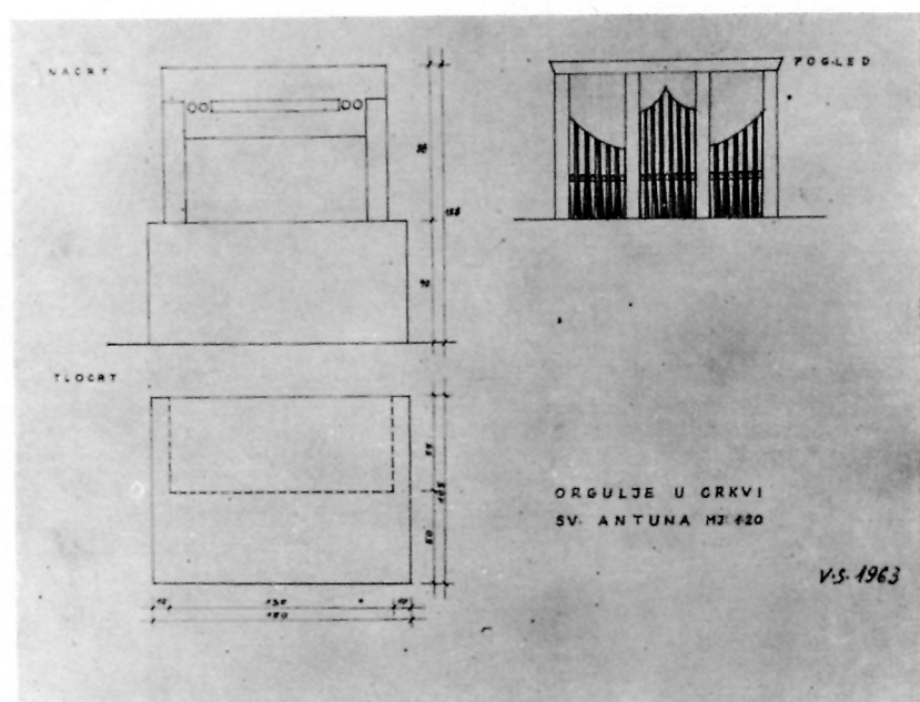
5 NACRT ORGULJA U KAPELI SV. ANTUNA U MATEINCIMA
