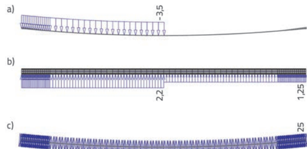
Slika 22. Neka opterećenja u uporabnoj kombinaciji K1 (stalni teret je automatski uključen, dok je prednapinjanje simulirano početnom deformacijom); a) Q_{0,5} - opterećenje pješacima preko pola raspona ( kN/m^2 ); b) W_{0,5} - pripadno vjetrovno opterećenje za Q_{0,5} ( kN/m ); c) \Delta T^* jednoliki prirast temperature ( ^{\circ}C )
