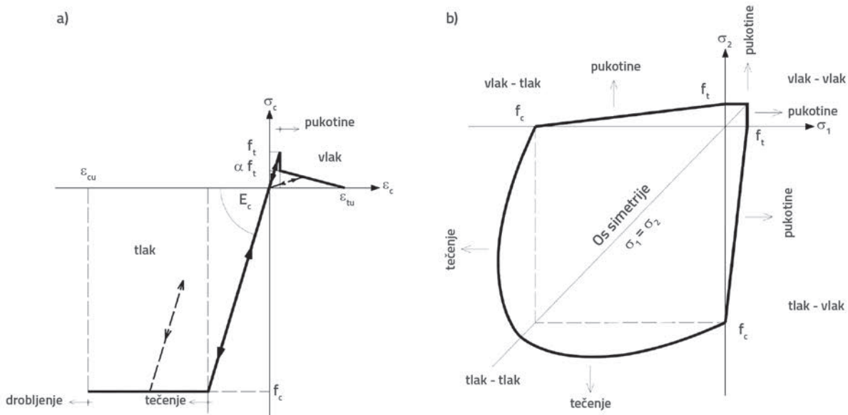
Slika 4. Grafički prikaz usvojenog modela ponašanja betona: a) jednodimenzionalni prikaz; b) 2D prikaz u polju glavnih napreznja
