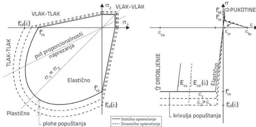
Slika 6. Grafički prikaz modela betona u uvjetima dinamičkog opterećenja: a) prikaz u polju glavnih naprezanja; b) jednodimenzionalni prikaz
