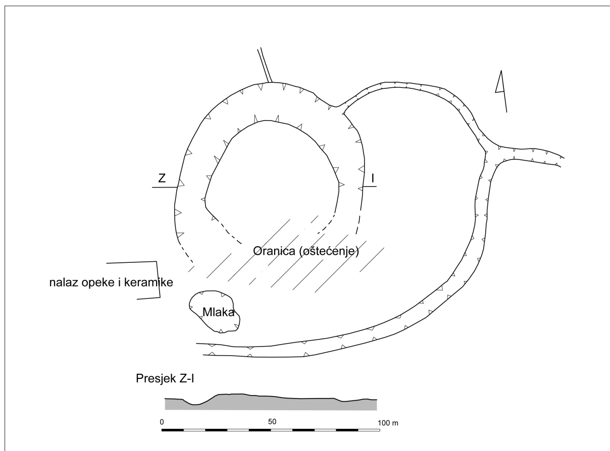
Sl. 10 Skica tlocrta gradišta Dijaneš – Dijaneško (crtež i izmjera: T. Tkalčec; digitalizacija: K. Jelinčić Vučković).
