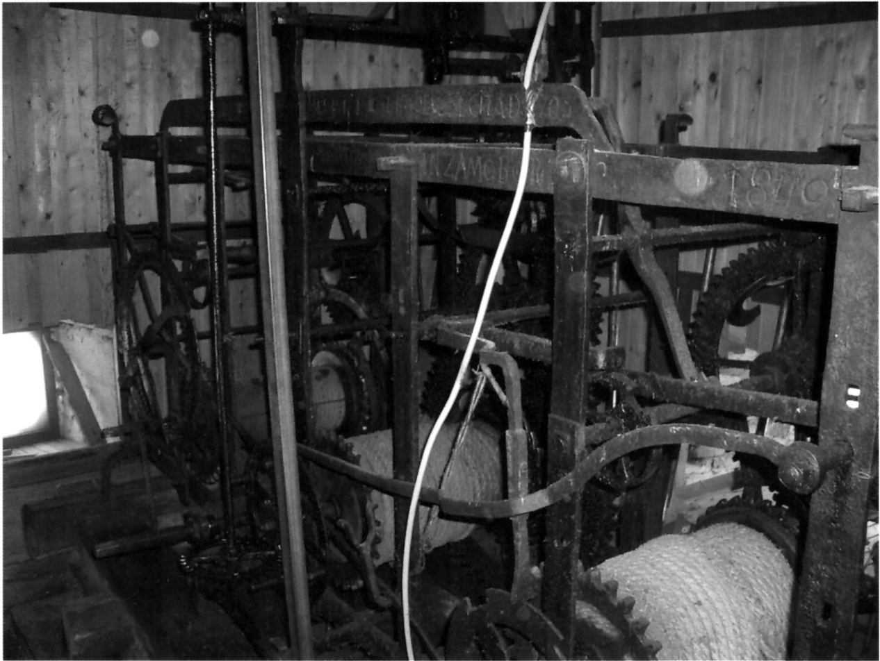
Satni mehanizam lepoglavskog sata
