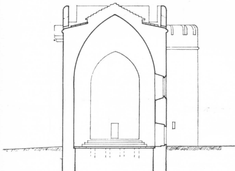
Vrboška, poprečni presjek broda crkve-tvrđave
