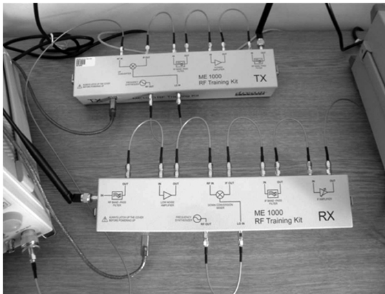
Slika 7. Edukacijski kit DreamCatcher (odašiljač, prijammik)
