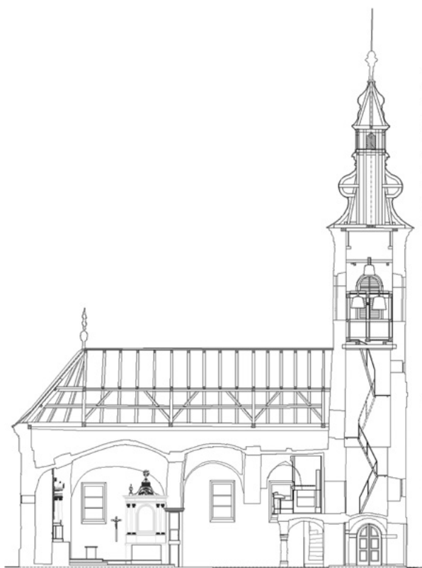
5. Kapela sv. Lovre, uzdužni presjek (planoteka KO u Varaždinu, izradila B. Petanjek) Chapel of St. Lawrence, longitudinal section (Plan Archive of the Conservation Department in Varaždin, drawing by B. Petanjek)
