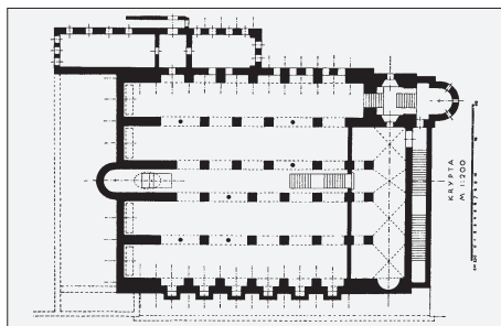
SL. 12. CRKVA MAJKE BOŽJE LURDSKE, PROJEKT ARHITEKTA JOŽE PLEČNIKA, TLOCRT KRIPTE
