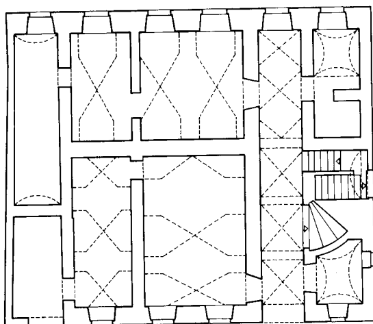
12. Tlocrt prizemlja kurije Kaptol 20
