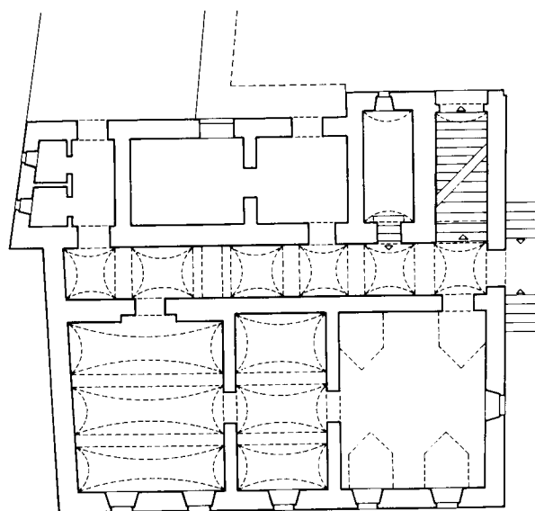
14. Tlocrt prizemlja kurije Kaptol 24
