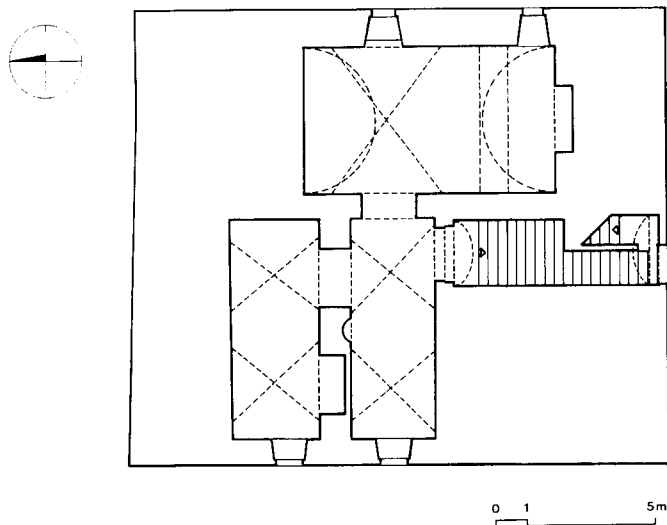
11. Tlocrt podruma kurije Kaptol 20
