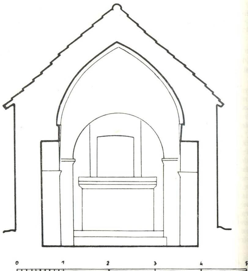
29. Žrnovnica, poprečni presjek crkve sv. Mihovila
