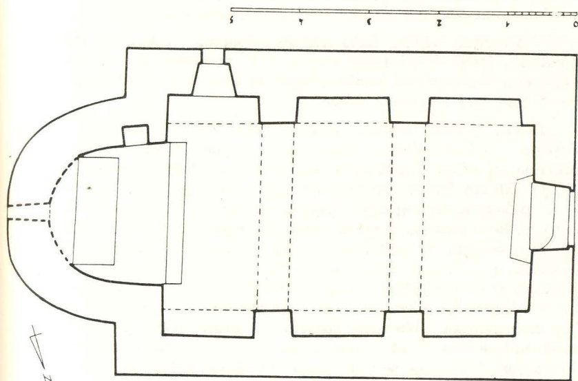
27. Žrnovnica, tlocrt crkve sv. Mihovila
