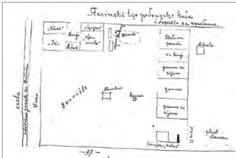
CRTEŽ »Starinski tip podravskè kuće i dvorišta sa zgradama« [37]
