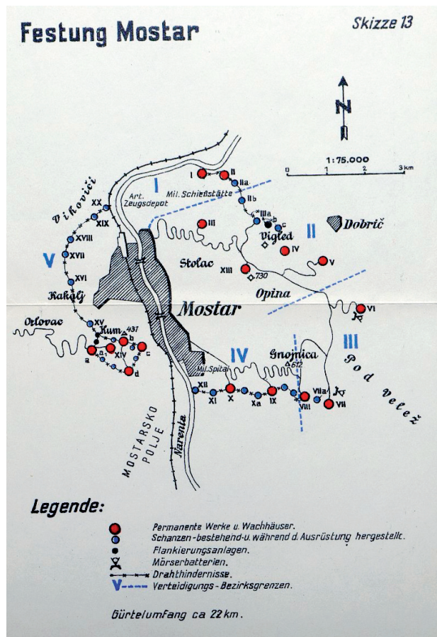
Plan pojaspne utvrde Mostar
