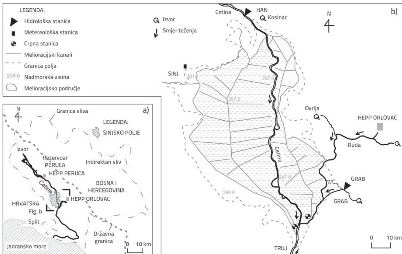
Slika 1. a) sliv rijeke Cetine; b) Sinjsko polje
