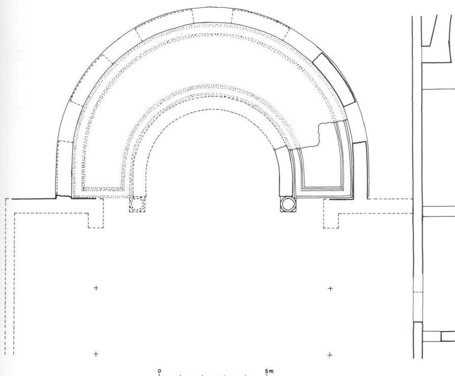
Tlocrt ostataka apsida starokršćanske katedrale u Zadru
