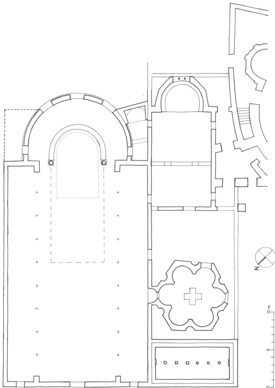
Grafička rekonstrukcija tlocrta katedrale s predromaničkim slojem građevina
