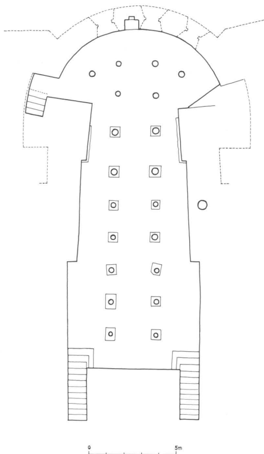
Tlocrt romaničke kripte katedrale u Zadru
