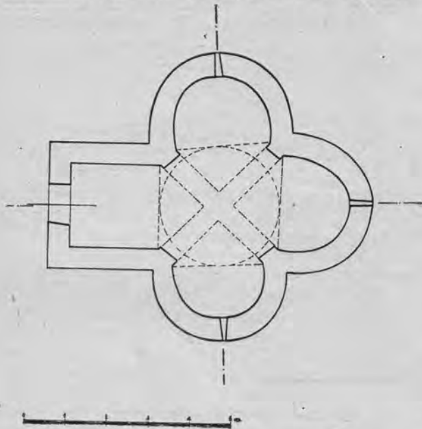
Sl. 7. — Tlocrt Sv. Krševana na Krku
