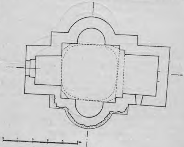
Sl. 6. — Tlocrt Sv. Donata na Krku
