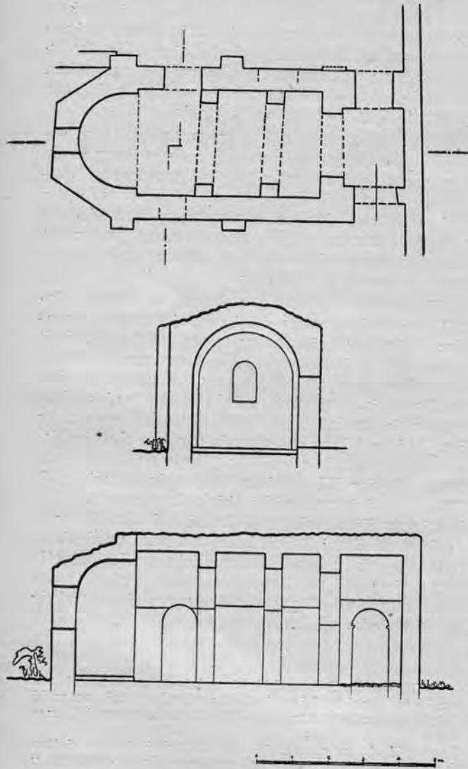
Sl. 12. — Sv. Mihovil na Limu, sjeverni objekt, tlocrt i presjeci
