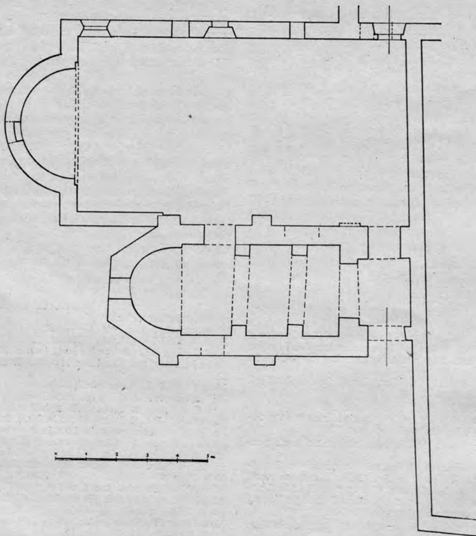
Sl. 11 — Tlocrt kompleksa Sv. Mihovila nad Limskom dragom
