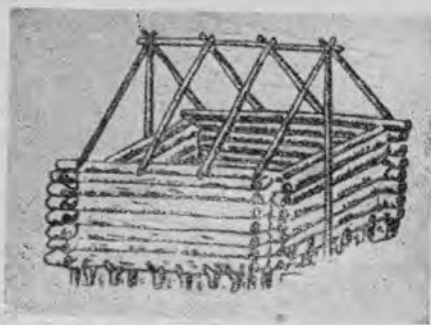
Sl. 4. — Konstrukcija krovišta stare slavenske nastambe u Parsecku (Po Korošcu prema Kostrzewskom)
