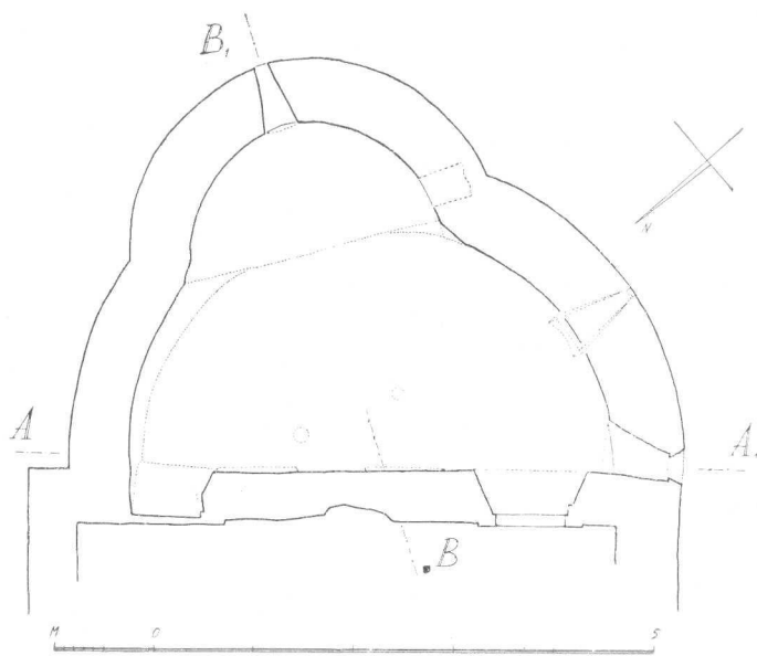
Sl. 3. Tlocrt ostataka stare kružne crkve sv. Marije u Malom Ižu
