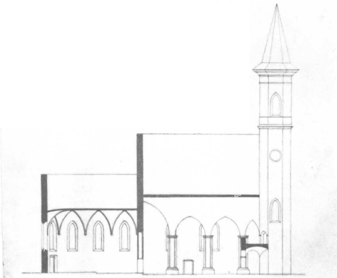
Sl. 6. Skica presjeka glogovničke crkve (planoteka Konzervatorskog Zavoda u Zagrebu, br. 596)
