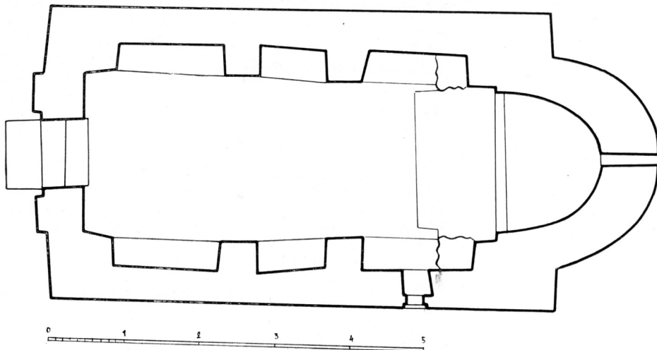
Tlocrt crkve sv. Jurja u Tučepima
