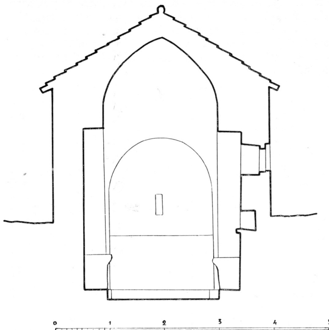
Presjek crkve sv. Jurja u Tučepima
