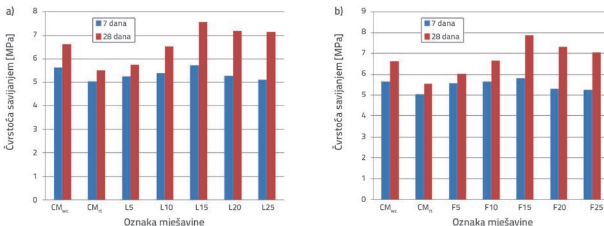
Slika 5. Čvrstoća savijanjem SCSCC betona: a) s dodatkom LECA agregata; b) s dodatkom FAA agregata
