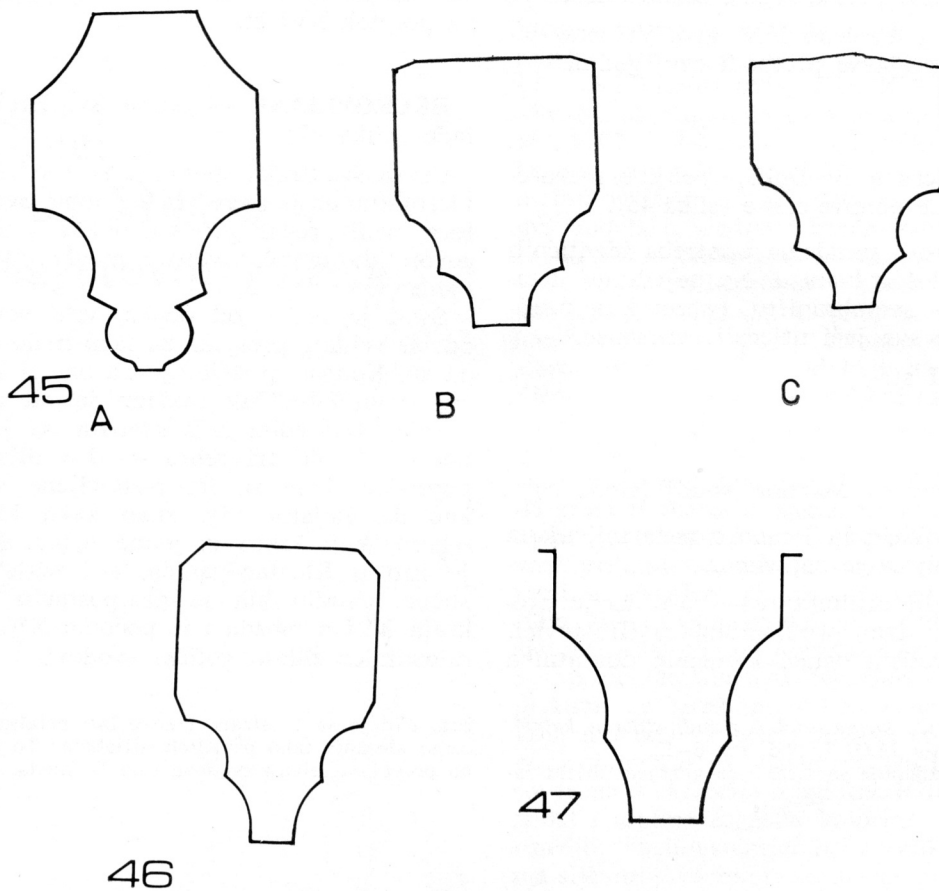
45 Hrastovica, crkva sv. Duha: spoliji rebara; 46 Prozorje, spolij rebra; 47 Brckovljani, crkva sv. Brcka
