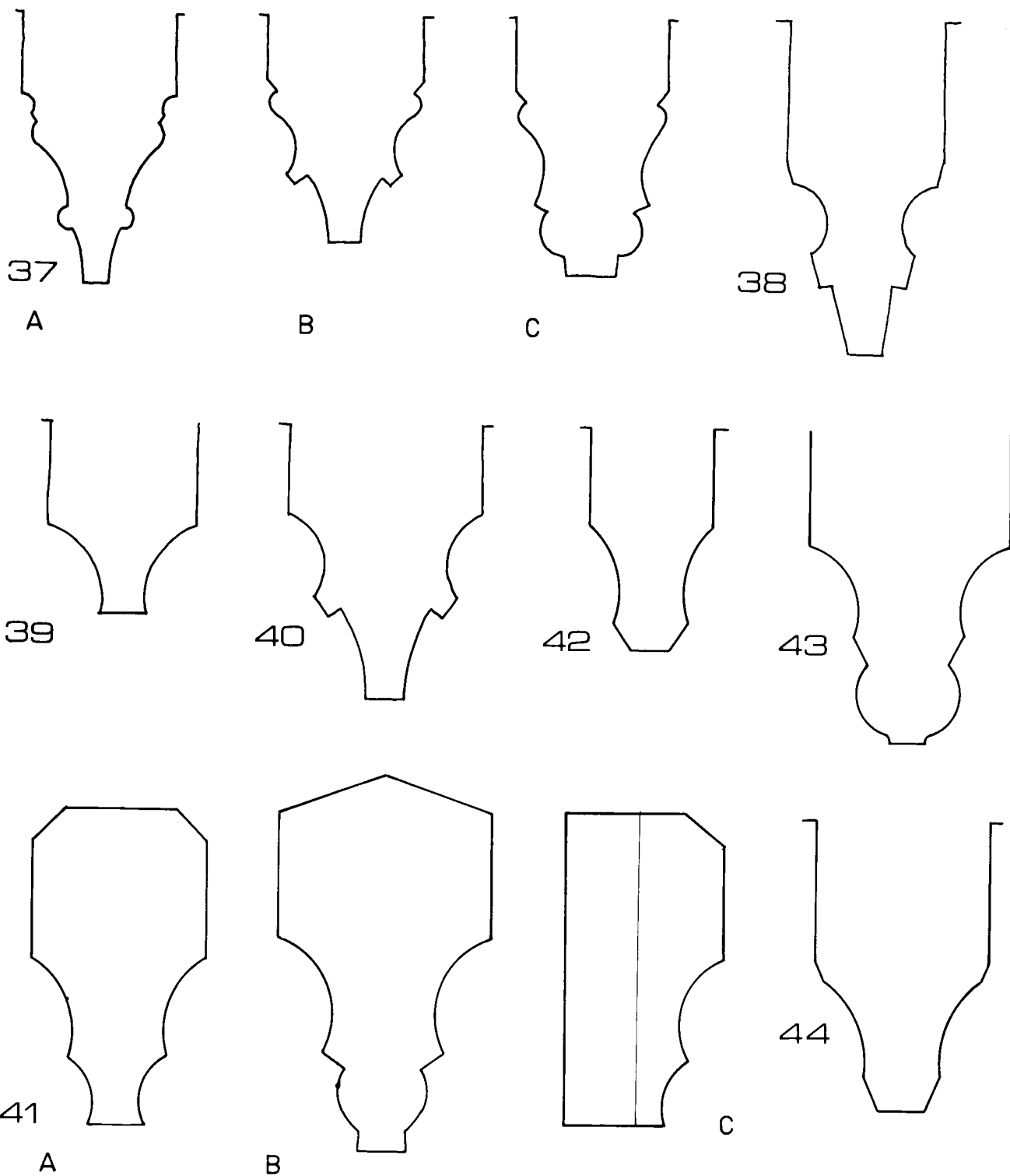
37 Voćin, bivša samostanska crkva — skice: a) rebra svoda istočne kapele, b) rebra klaustura i lađe, c) rebra iz svetišta; 38 Nova Rača, skica rebra svoda ispod tornja; 39 Tomaš, skica rebra iz kapele sv. Tome; 40 Zagreb, skica rebra iz lađe katedrale; 41 Kloštar Ivanić, crkva franjevačkog samostana: a) diagonalna rebra svetišta, b) poprečna rebra svetišta, c) polurebro; 42 Klenovnik, crkva sv. Vuka; 43 Dubrava, crkva sv. Martina; 44 Kalnik, crkva sv. Brcka
