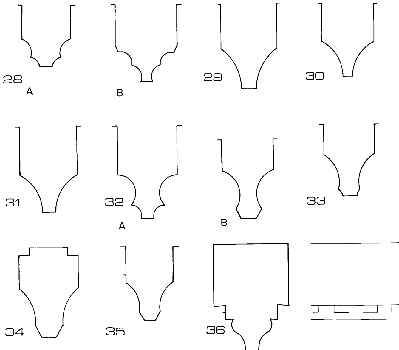
28 Markuševac, župna crkva: a) rebro kapele, b) rebro svetišta; 29 Tuhelj, župna crkva; 30 Krašić, župna crkva; 31 Petrovina, župna crkva; 32 Remetinec, župna crkva: a) rebro iz lađe, b) rebro svoda ispod tornja; 33 Bedenica, župna crkva; 34 Očura, kapela sv. Jakova; 35 Belec, crkva sv. Jurja, rebro svoda ispod tornja; 36 Ružica, rebro iskopano prilikom zaštitnih radova
