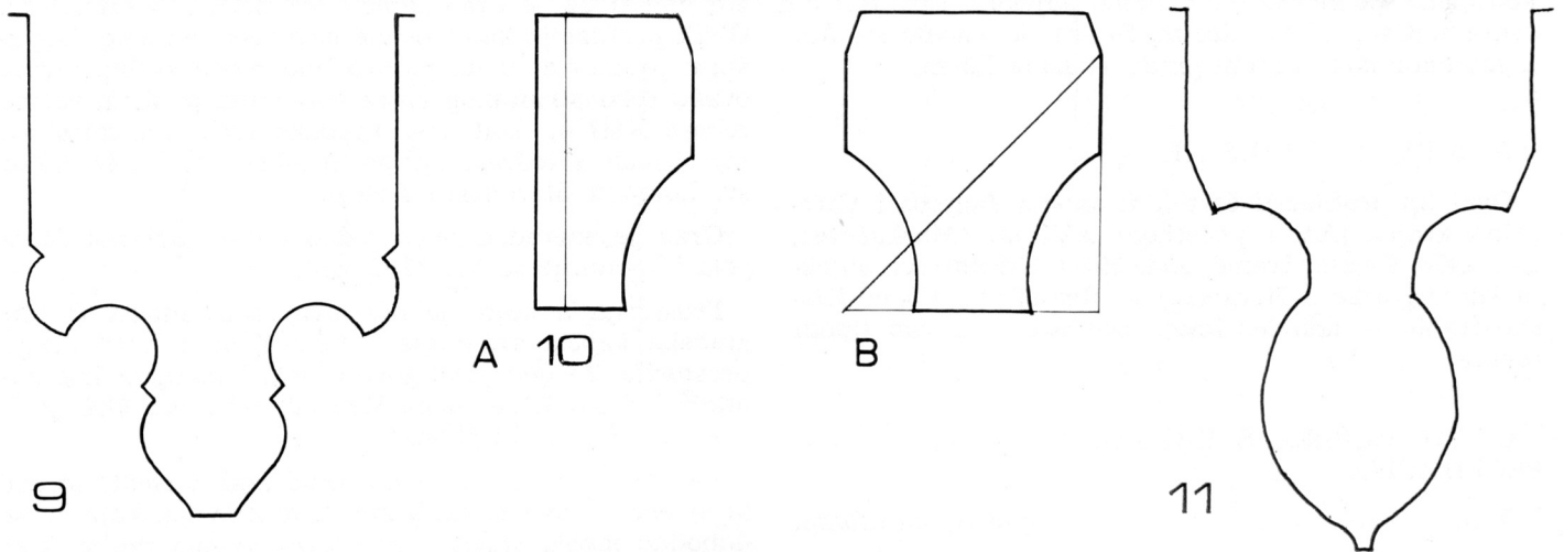
9 Slavonska Požega, crkva sv. Lovre; 10 Grebengrad, a) polurebro, b) rekonstrukcija rebra; 11 Topusko, skica rebra glavne lađe
