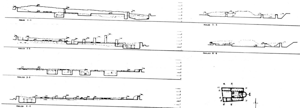
9 Projekt konzervacije, rekonstrukcije i prezentacije — presjeci
