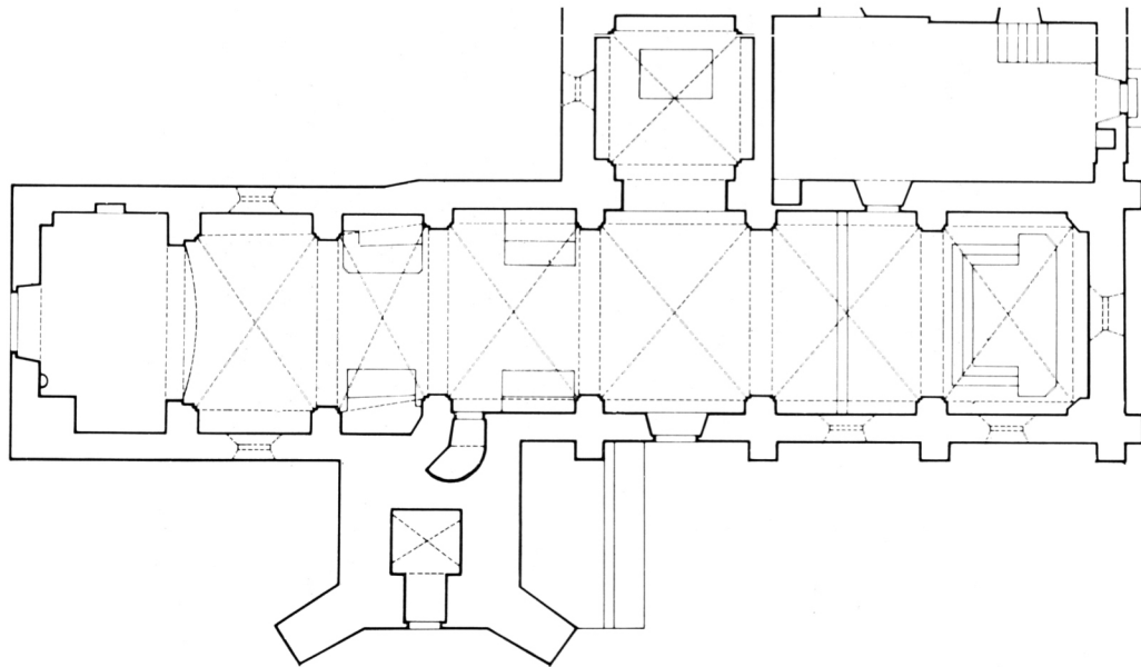
6 Gora, Crkva uzašašća Bl. Dj. Marije — Tlocrt današnjeg stanja. Snimak ing. arh. Sonja Pinter
